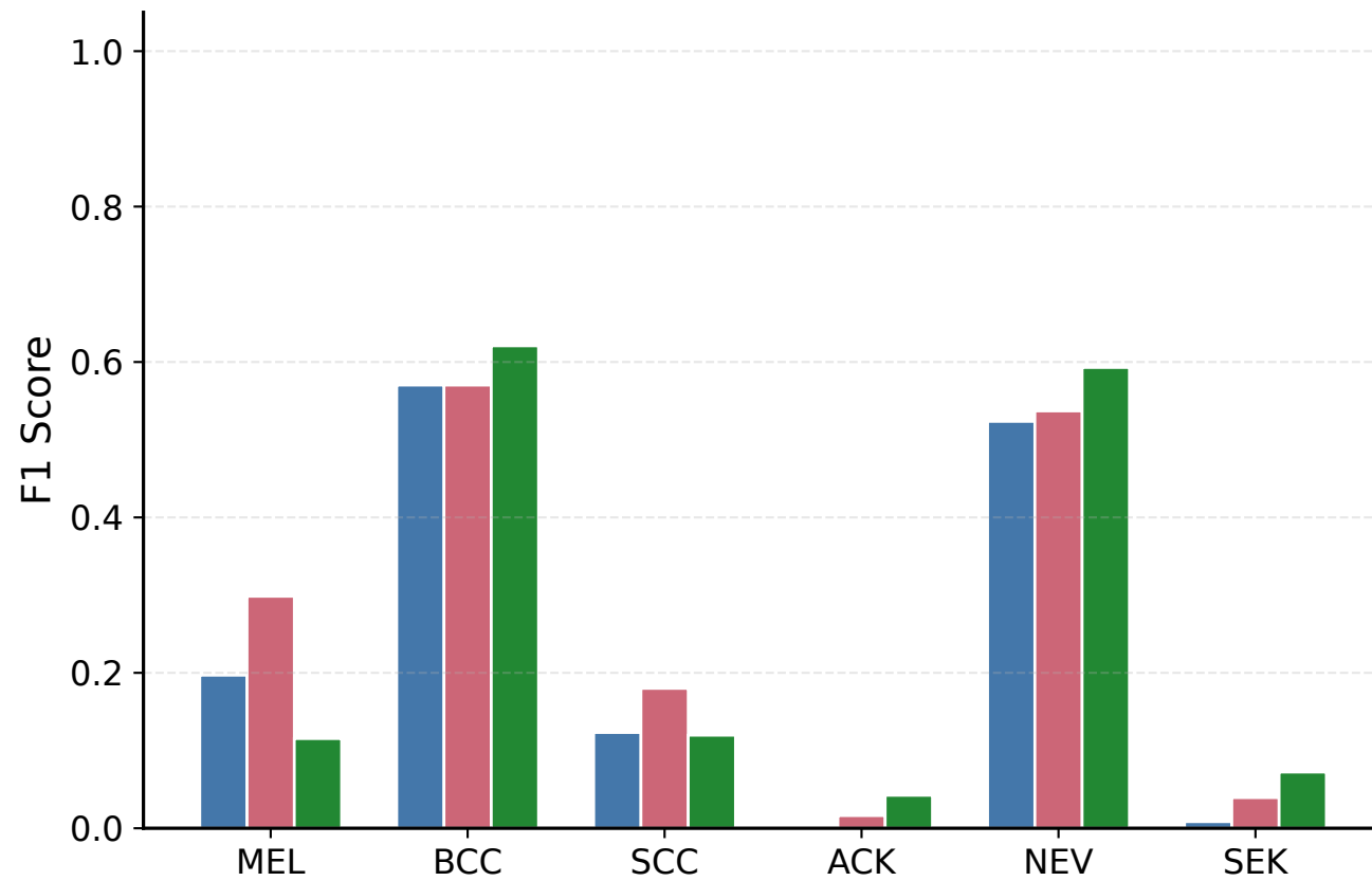
F1 Score
