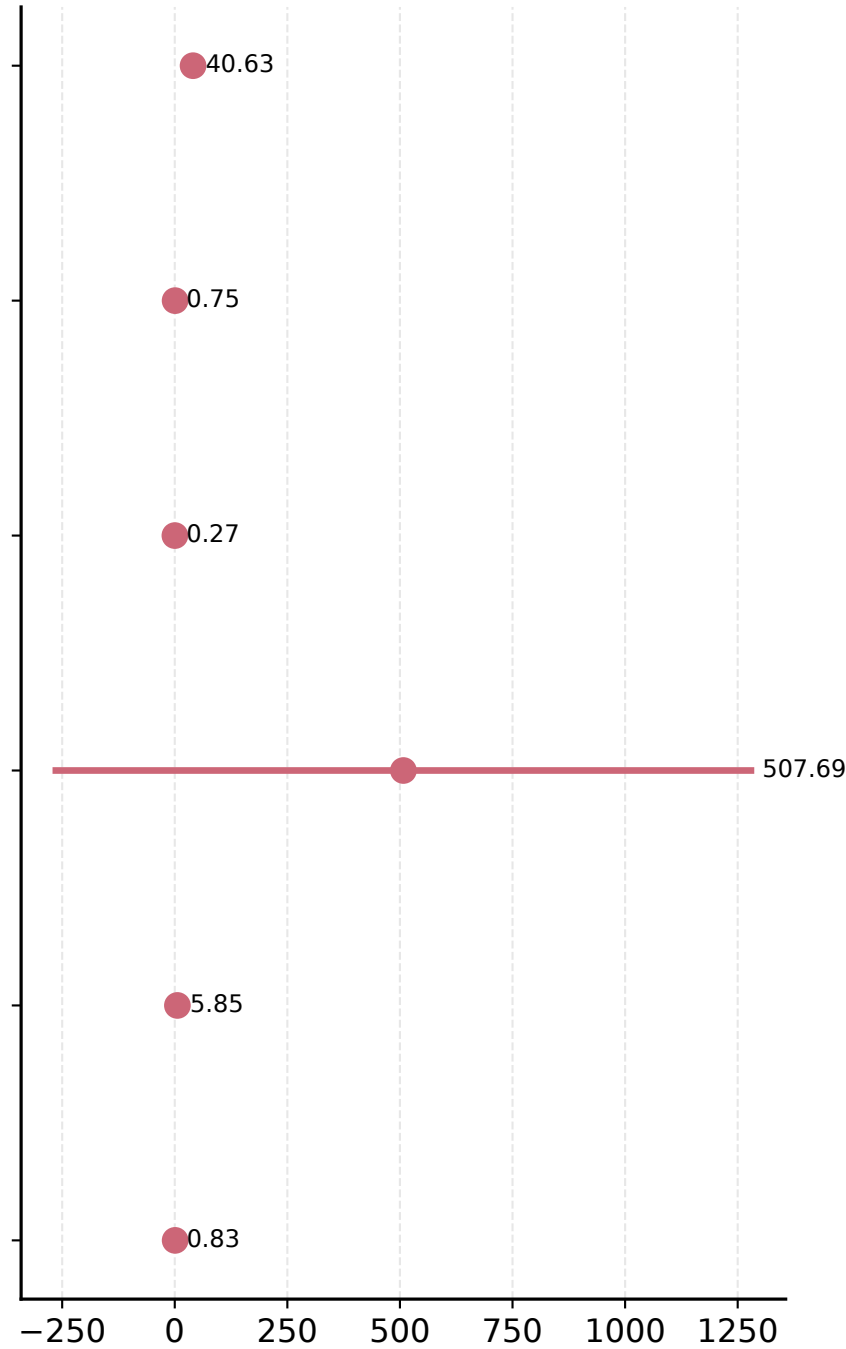
GMU
