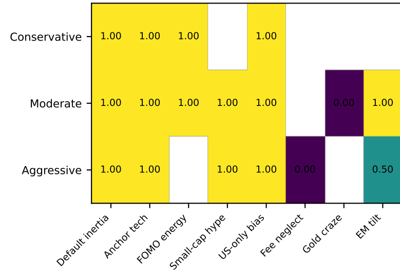
gemini-2.5-flash
