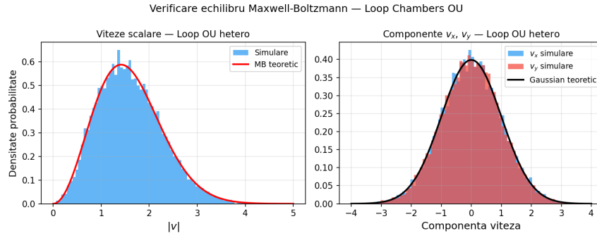
Figura 9: Distribuția modulului vitezei în loop_chambers cu OUBounce eterogen față de curba Maxwell–Boltzmann teoretică. Distribuția marginală a vitezelor e corectă, dar aceasta nu garantează singură echilibrul termodinamic global.
