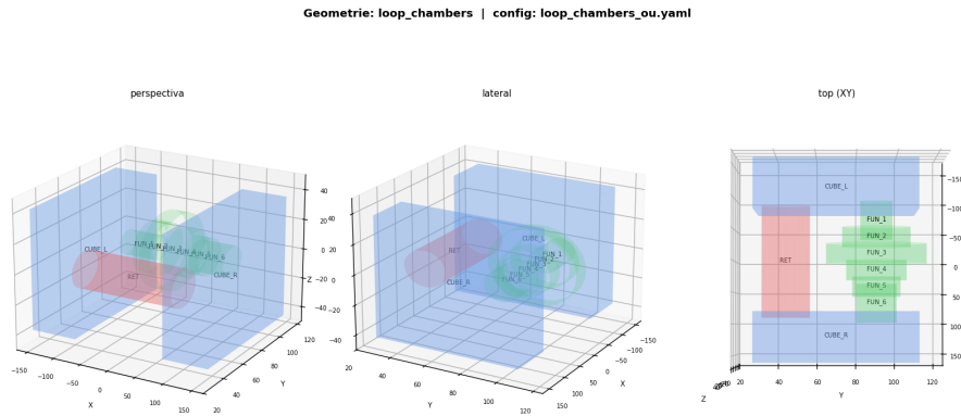
Figura 5: Vedere perspectivă a geometriei loop_chambers : camerele CUBE_L (stânga) și CUBE_R (dreapta) sunt conectate prin canalul cu pâlnie (sus) și canalul de retur RET (jos). Culoarele diferite indică piesele geometrice cu materiale distincte.
