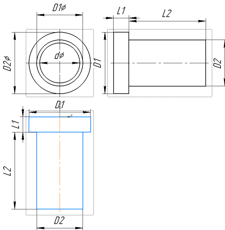
Рисунок 2.1 — Модель ступенчатой втулки
