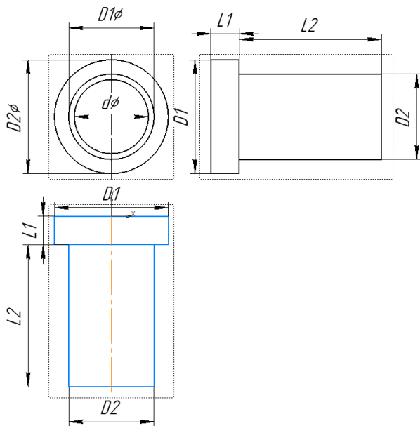
Рисунок 2.1 — Модель ступенчатой втулки
