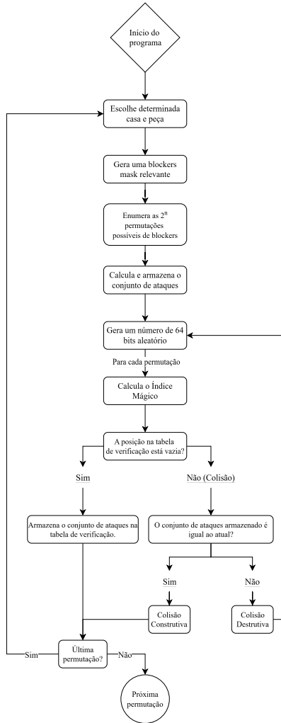
Figura 2: Geração e validação de um número mágico
