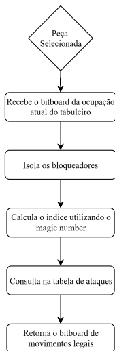
Figura 3: Consulta de ataques em tempo de execução com magic bitboards
