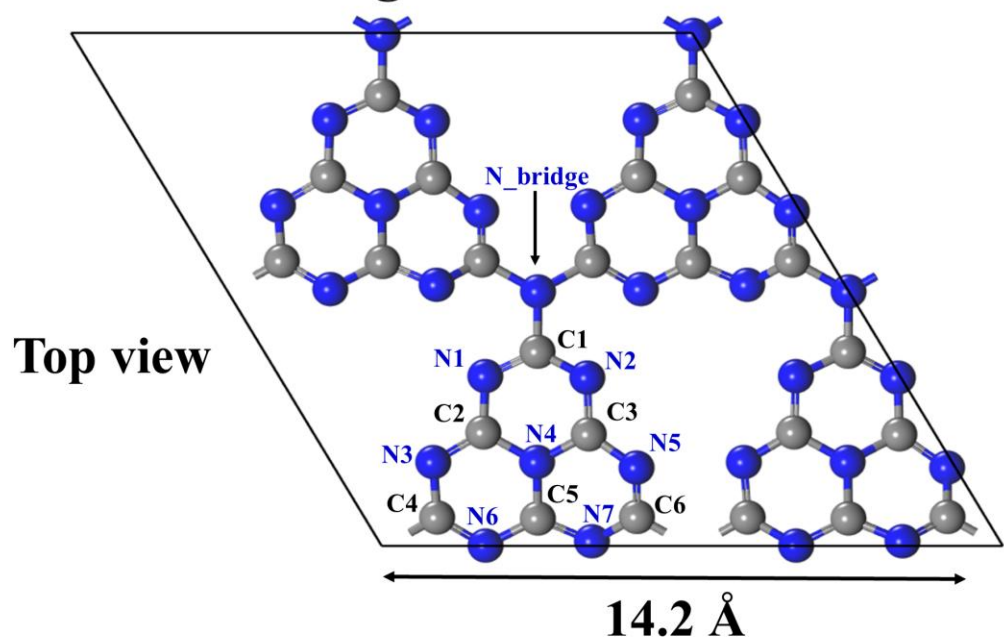
a) Planar g-C 3 N 4
