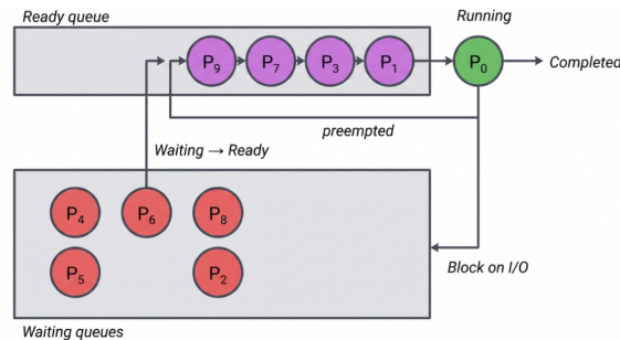
Figura 5. Diagrama de funcionamento do Round-Robin [da Costa 2026]
