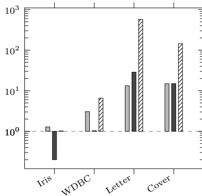
(b) Predição
