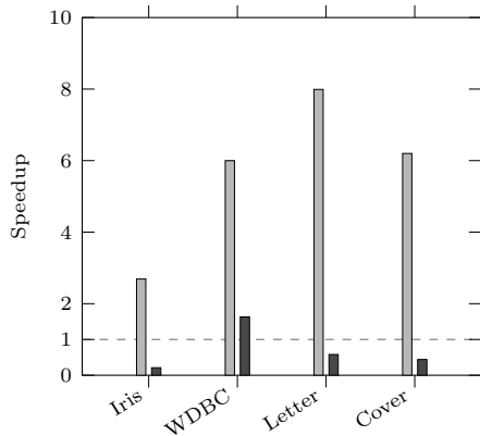
(a) Treino
