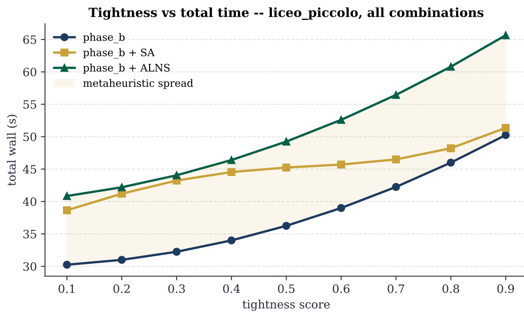
FIGURA 24.7 – Tempo totale vs tightness dello scenario, per le tre combinazioni dominanti (Phase B puro, + SA, + ALNS). La banda avorio è la dispersione delle metaeuristiche: aumenta con la tightness, segno che gli scenari più stretti beneficiano di più esplorazione.
