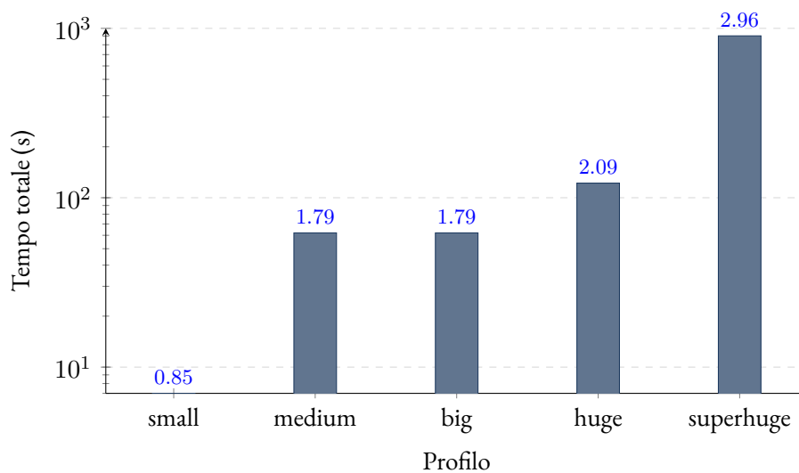
FIGURA B.1 – Tempo totale della pipeline (scala logaritmica). Si nota la salita lineare in scala log fino a huge, con il salto previsto su superhuge dovuto alla dimensione del Phase A.
