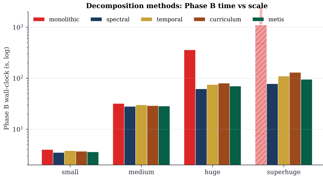
FIGURA 24.2 – Wall-clock di Phase B per metodo di decomposizione, su quattro scale (small, medium, huge, superhuge). La modalità monolitica va in timeout su superhuge; le quattro decomposizioni convergono in tempo paragonabile, con un leggero vantaggio per spectral e metis sui regimi grandi. Scala logaritmica per contenere la dispersione fra small e superhuge.
