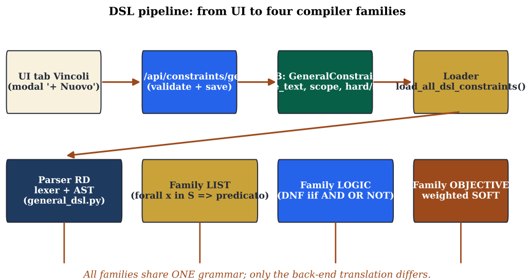
FIGURA 23.3 – Architettura del DSL generico: stessa grammatica e stesso AST, quattro back-end di traduzione. La differenza fra “valutare una soluzione” (evaluator post-hoc) e “costruire un modello” (compiler verso CP-SAT) si traduce in due attraversamenti diversi dello stesso albero.
