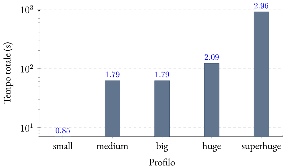
FIGURA 29.1 – Tempo totale della pipeline (scala logaritmica). Si nota la salita lineare in scala log fino a huge, con il salto previsto su superhuge dovuto alla dimensione del Phase A.
