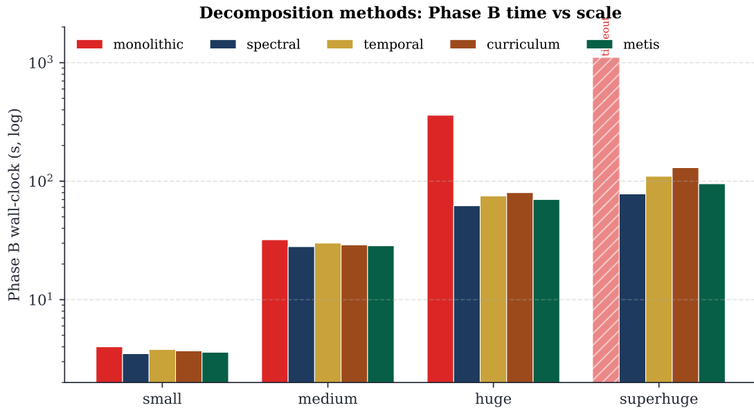
FIGURA 23.2 – Wall-clock di Phase B per metodo di decomposizione, su quattro scale (small, medium, huge, superhuge). La modalità monolitica va in timeout su superhuge; le quattro decomposizioni convergono in tempo paragonabile, con un leggero vantaggio per spectral e metis sui regimi grandi. Scala logaritmica per contenere la dispersione fra small e superhuge.
