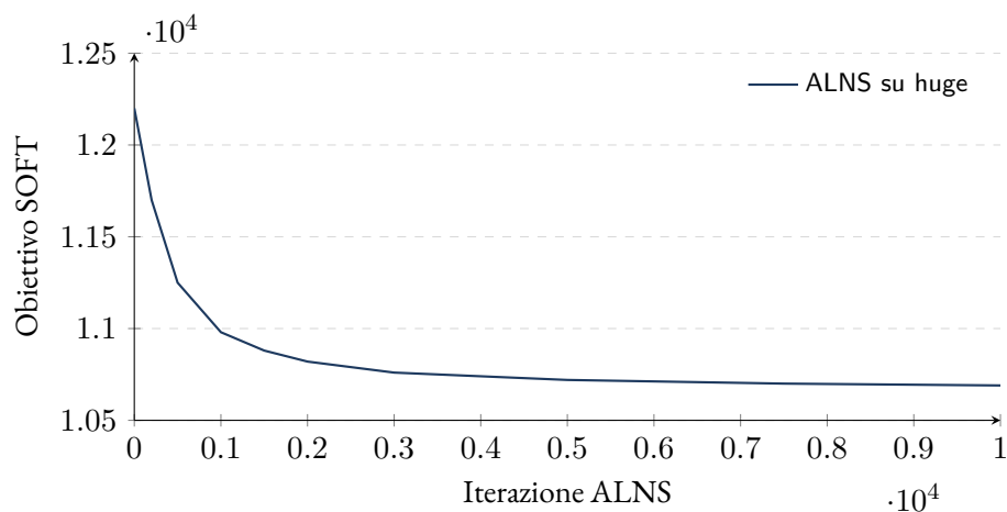
Figura B.3: Convergenza di ALNS sul profilo huge: il miglioramento si concentra nei primi 1000–2000 step e poi satura, tipico delle metaeuristiche.
