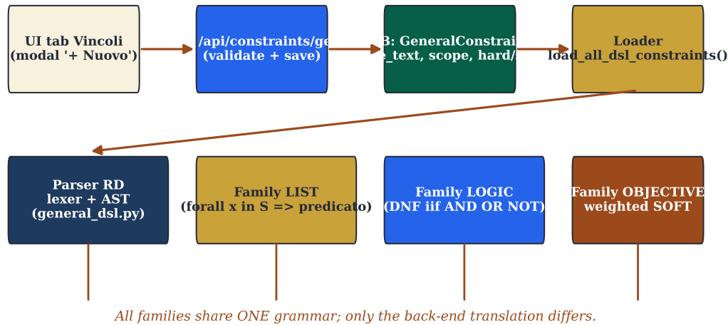
FIGURA 21.2 – Pipeline del DSL: dal modal nell’UI fino alle quattro famiglie di backend. Il pulsante validate attiva solo il parser (e ritorna gli errori in tempo reale); il save attiva il loop completo: persistenza in constraints_general , ricarica al successivo POST /api/optimize , valutazione post-hoc al termine.
