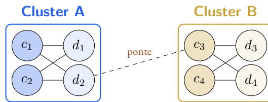
FIGURA 11.1 – Esempio di grafo bipartito con due cluster naturali e un “ponte” debole. Il vettore di Fiedler assegna componenti di segno opposto ai due cluster.
