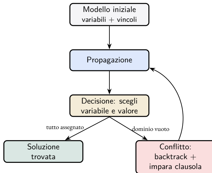
FIGURA 10.1 – Il ciclo di funzionamento di CP-SAT. Dopo aver propagato il modello iniziale, il solver alterna decisioni e propagazioni; ogni conflitto produce una clausola appresa che evita di ripetere lo stesso errore.
