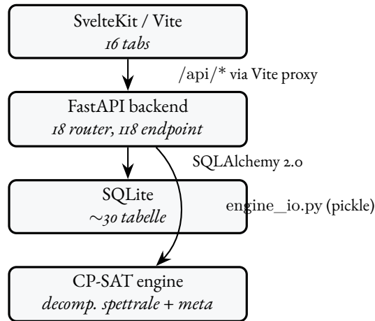
FIGURA 19.1 – Architettura a blocchi della webapp.
