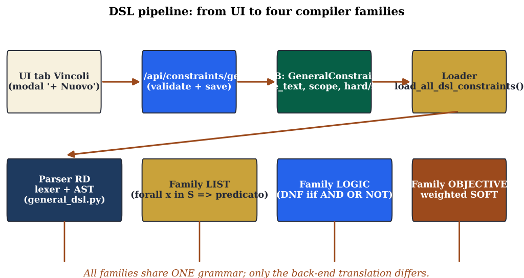
FIGURA 21.3 – Architettura del DSL generico: stessa grammatica e stesso AST, quattro back-end di traduzione. La differenza fra “valutare una soluzione” (evaluator post-hoc) e “costruire un modello” (compiler verso CP-SAT) si traduce in due attraversamenti diversi dello stesso albero.
