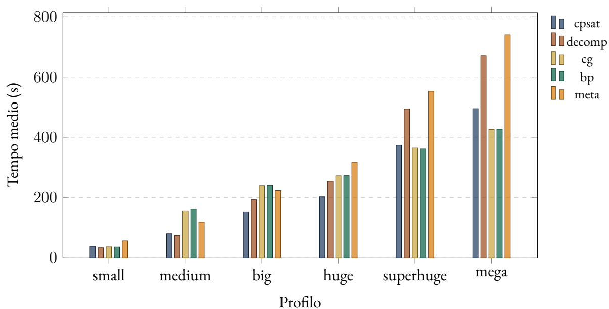
FIGURA 28.8 – Tempo medio in secondi per famiglia di tecnica e profilo. Le celle in stato non-OK (unwired, timeout, exception) sono escluse dal calcolo. Il bar chart resta vuoto per le combinazioni famiglia-profilo prive di celle riuscite.
