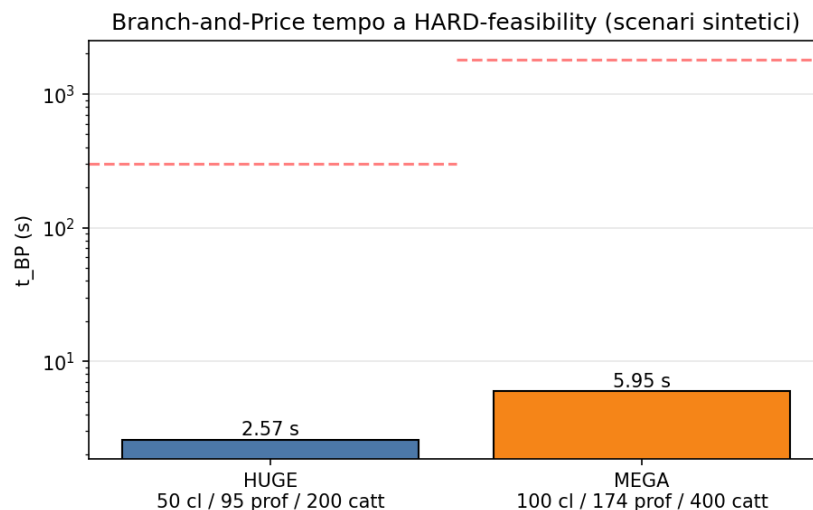
FIGURA 28.4 – Tempo di convergenza del Branch-and-Price (scala logaritmica). Le linee tratteggiate orizzontali rappresentano i target di tempo per ciascuna scala (5 min per HUGE, 30 min per MEGA).
