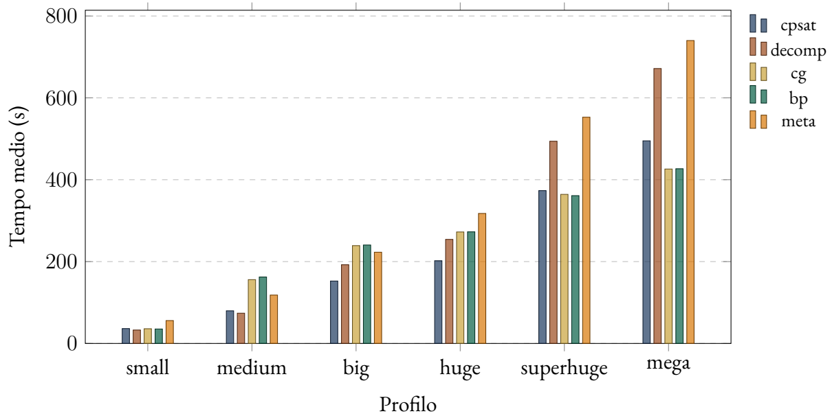
FIGURA 28.6 – Tempo medio in secondi per famiglia di tecnica e profilo. Le celle in stato non-OK (unwired, timeout, exception) sono escluse dal calcolo. Il bar chart resta vuoto per le combinazioni famiglia-profilo prive di celle riuscite.
