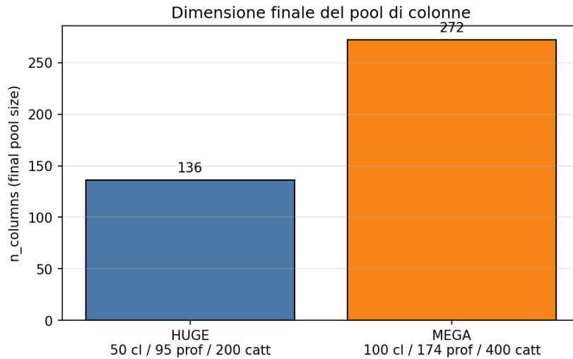
FIGURA 28.5 – Dimensione finale del pool di colonne dopo il loop Branch-and-Price.
