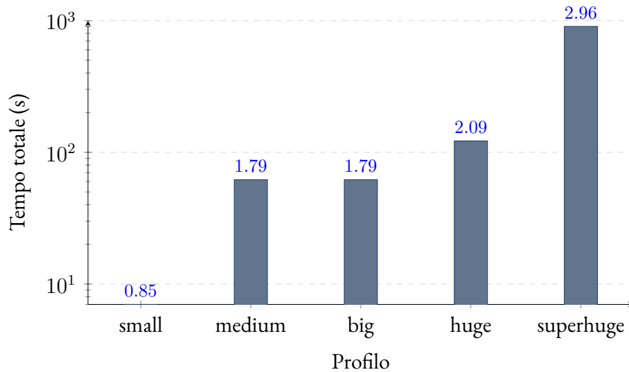
FIGURA 29.1 – Tempo totale della pipeline (scala logaritmica). Si nota la salita lineare in scala log fino a huge, con il salto previsto su superhuge dovuto alla dimensione del Phase A.
