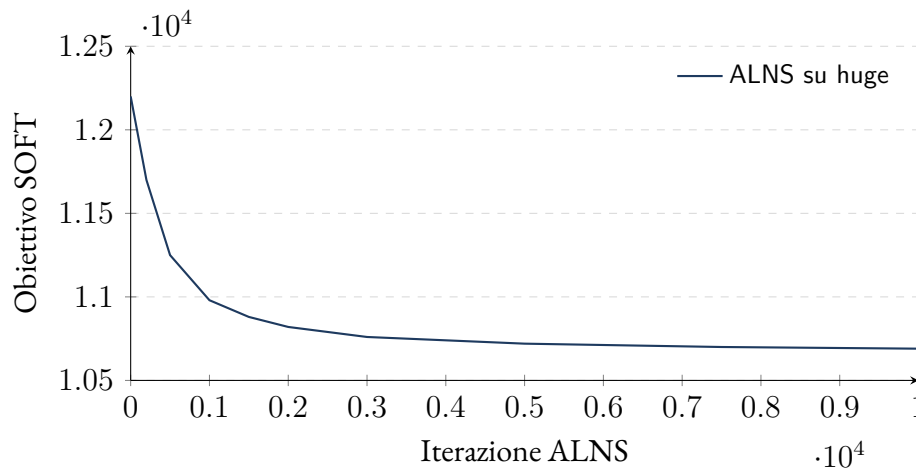
FIGURA 29.3 – Convergenza di ALNS sul profilo huge: il miglioramento si concentra nei primi 1000–2000 step e poi satura, tipico delle metaeuristiche.
