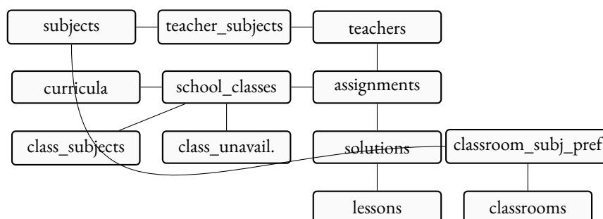
FIGURA 8.1 – Relazioni rilevanti del modello dati (semplificato).
