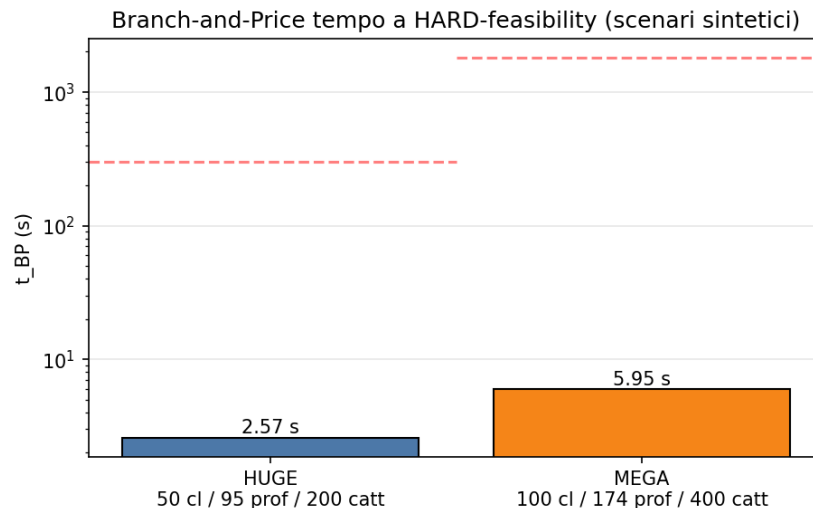
FIGURA 29.4 – Tempo di convergenza del Branch-and-Price (scala logaritmica). Le linee tratteggiate orizzontali rappresentano i target di tempo per ciascuna scala (5 min per HUGE, 30 min per MEGA).
