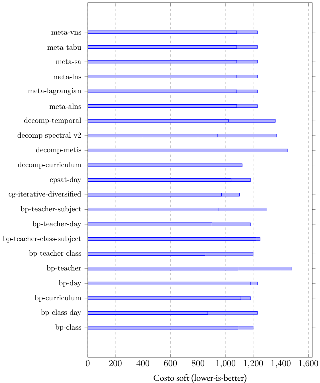
FIGURA 29.9 – Costo finale (soft objective) per tecnica sul profilo small. Le tecniche sono in ordine di apparizione nel CSV: leggile dall’alto al basso per il cluster cpsat-decomp-cg-bp-meta.
