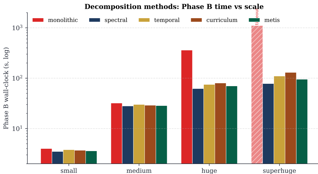
FIGURA 23.2 – Wall-clock di Phase B per metodo di decomposizione, su quattro scale (small, medium, huge, superhuge). La modalità monolithic va in timeout su superhuge; le quattro decomposizioni convergono in tempo paragonabile, con un leggero vantaggio per spectral e metis sui regimi grandi. Scala logaritmica per contenere la dispersione fra small e superhuge.
