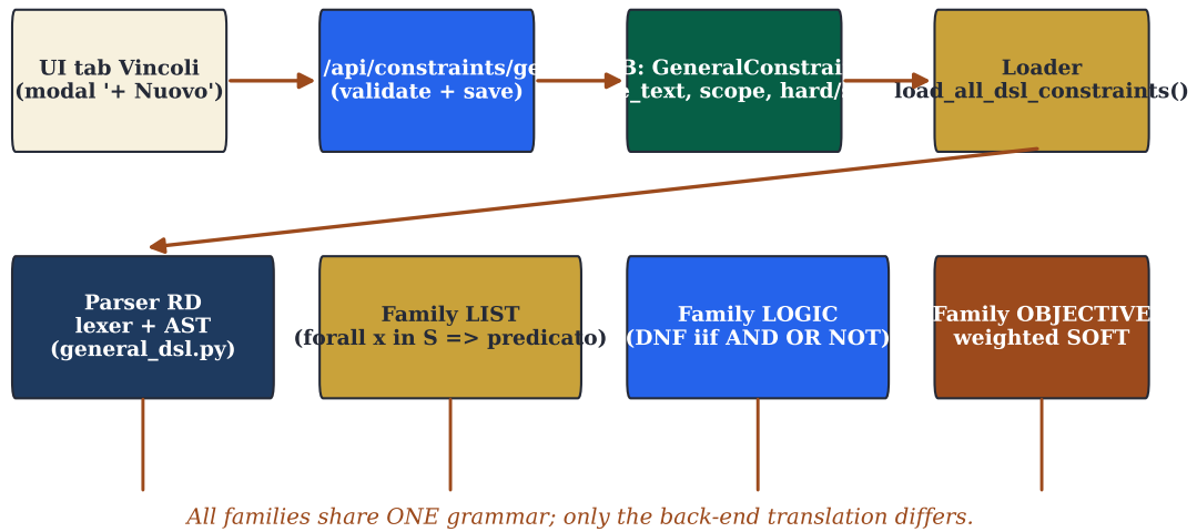
FIGURA 13.3 – Architettura del DSL generico: stessa grammatica e stesso AST, quattro back-end di traduzione. La differenza fra “valutare una soluzione” (evaluator post-hoc) e “costruire un modello” (compiler verso CP-SAT) si traduce in due attraversamenti diversi dello stesso albero.
