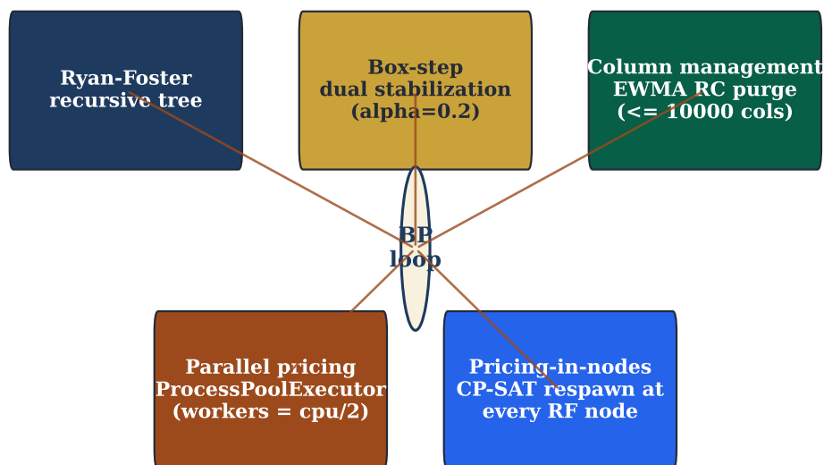
FIGURA 23.3 – Le cinque tecniche scalabili che si compongono attorno al loop Branch-and-Price: Ryan-Foster recursive tree, box-step dual stabilization, column management, parallel pricing, pricing-in-nodes (Step 4). Tutte e cinque sono attive di default in mode="branch-and-price" ; ciascuna può essere disabilitata via flag.
