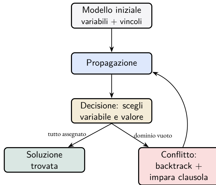
FIGURA 15.1 – Il ciclo di funzionamento di CP-SAT. Dopo aver propagato il modello iniziale, il solver alterna decisioni e propagazioni; ogni conflitto produce una clausola appresa che evita di ripetere lo stesso errore.
