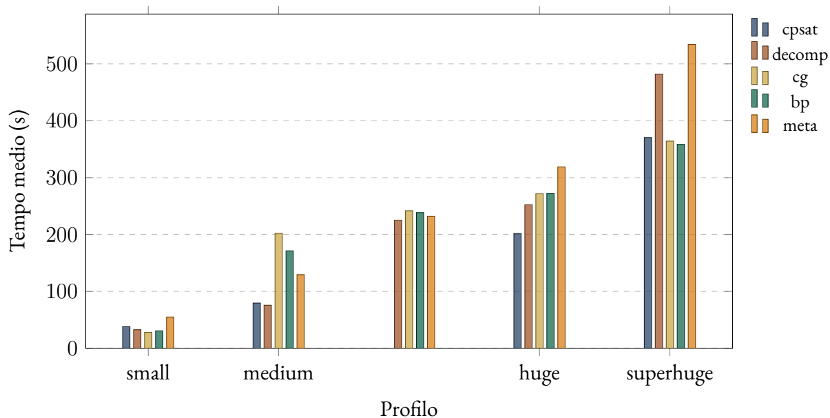
FIGURA 29.10 – Tempo medio in secondi per famiglia di tecnica e profilo. Le celle in stato non-OK (unwired, timeout, exception) sono escluse dal calcolo. Il bar chart resta vuoto per le combinazioni famiglia-profilo prive di celle riuscite.
