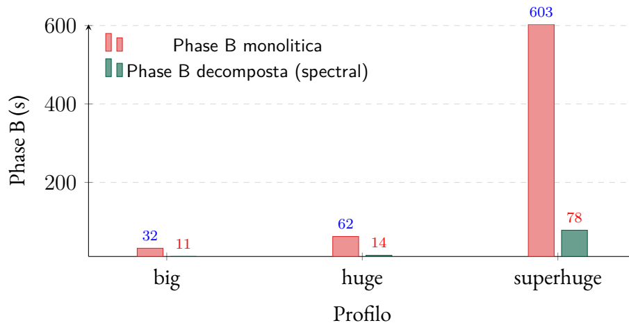
FIGURA 29.2 – Confronto del tempo di Phase B con e senza decomposizione spettrale, sui profili medio-grandi.
