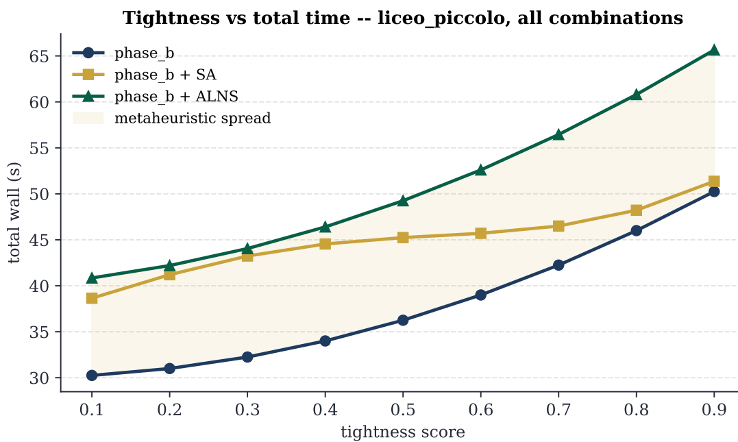
FIGURA 23.7 – Tempo totale vs tightness dello scenario, per le tre combinazioni dominanti (Phase B puro, + SA, + ALNS). La banda avorio è la dispersione delle metaeuristiche: aumenta con la tightness, segno che gli scenari più stretti beneficiano di più esplorazione.
