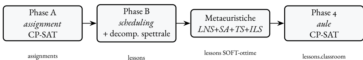
FIGURA 14.1 – Pipeline a 4 fasi.
