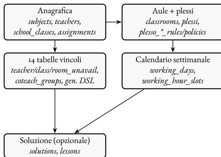
FIGURA 9.1 – Anatomia di <profilo>.sqlite: cinque blocchi tematici, tutti popolati da build_profile_db.py con seed deterministico.
