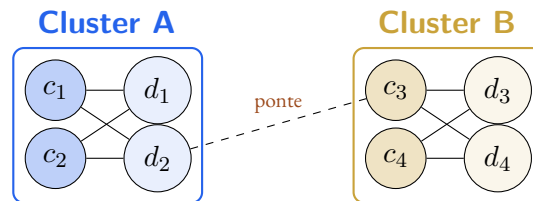
FIGURA 17.1 – Esempio di grafo bipartito con due cluster naturali e un “ponte” debole. Il vettore di Fiedler assegna componenti di segno opposto ai due cluster.
