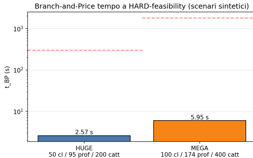
FIGURA 27.4 – Tempo di convergenza del Branch-and-Price (scala logaritmica). Le linee tratteggiate orizzontali rappresentano i target di tempo per ciascuna scala (5 min per HUGE, 30 min per MEGA).
