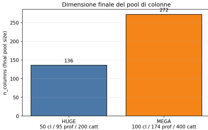
FIGURA 27.5 – Dimensione finale del pool di colonne dopo il loop Branch-and-Price.
