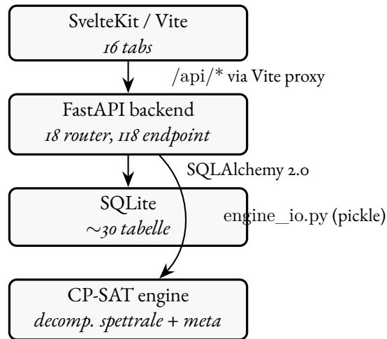
FIGURA A.1 – Architettura a blocchi della webapp.
