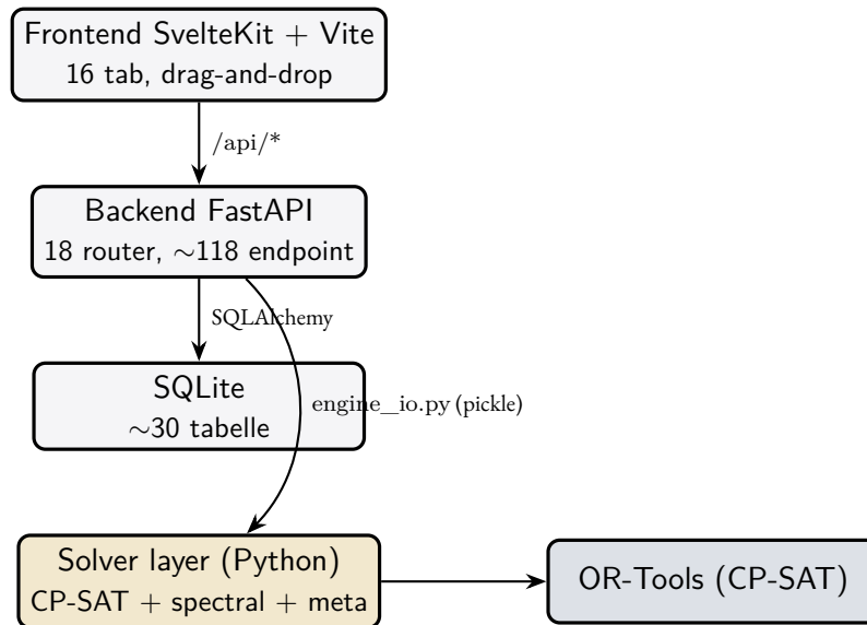
FIGURA 1.1 – Architettura a blocchi di \pi Tantum: il frontend parla al backend tramite REST, il backend persiste su SQLite e dialoga con il solver attraverso un convertitore esplicito basato su pickle, il solver invoca OR-Tools per le risoluzioni CP-SAT.
