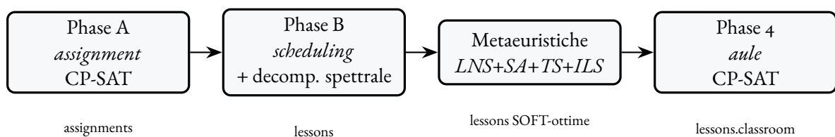
FIGURA 13.1 – Pipeline a 4 fasi.
