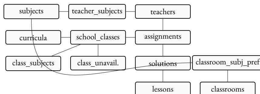
FIGURA 7.1 – Relazioni rilevanti del modello dati (semplificato).
