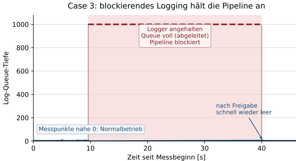
Abbildung 2: Log-Queue bei angehaltenem Logger. Die schattierte Phase enthält keine Messpunkte, weil der Logger-Prozess samt Mess-Thread pausiert. Aus dem anschließenden Rücksprung lässt sich ableiten, dass die Queue in dieser Phase vollgelaufen ist.
