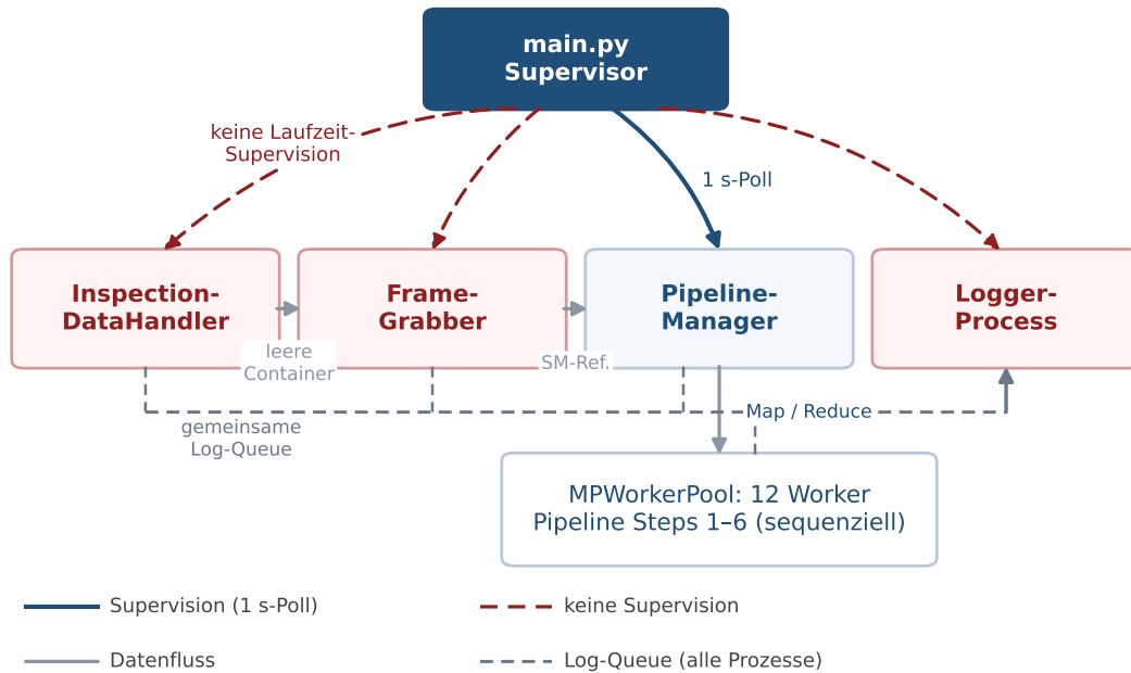
Abbildung 1: Prozess-Topologie von ROSI. main.py überwacht zur Laufzeit nur den PipelineManager (1 s-Poll); die drei rot markierten Service-Prozesse laufen ohne Laufzeit-Supervision (Case 1). Graue Pfeile zeigen den Datenfluss; große Bilddaten wandern nicht durch die Queues, sondern als Shared-Memory-Referenzen. Alle Prozesse loggen über die gemeinsame Log-Queue.
