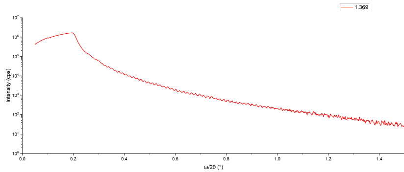
(d) 1.369 kÅ SiO 2 thin film
