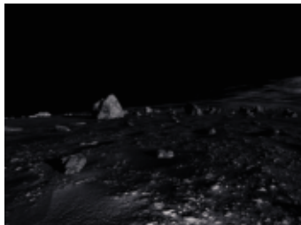
RGB
