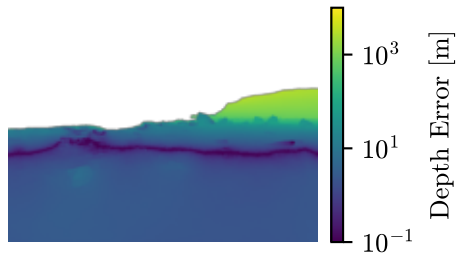
Depth Pro
