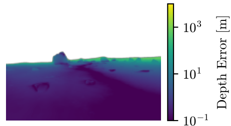
DPT
