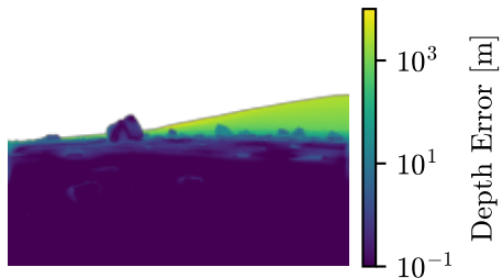
RAFTStereo
