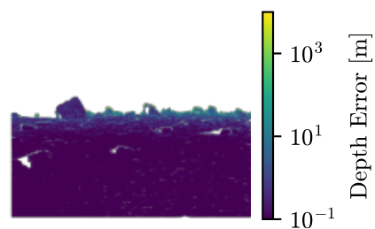
BM
