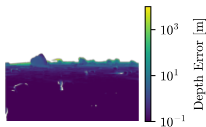
SGBM
