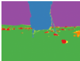
Unet
