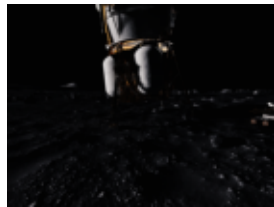
RGB
