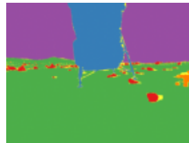
Segformer
