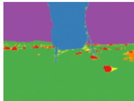
DeepLabV3
