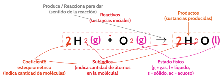
Figura 5: Anatomía de una ecuación química.
