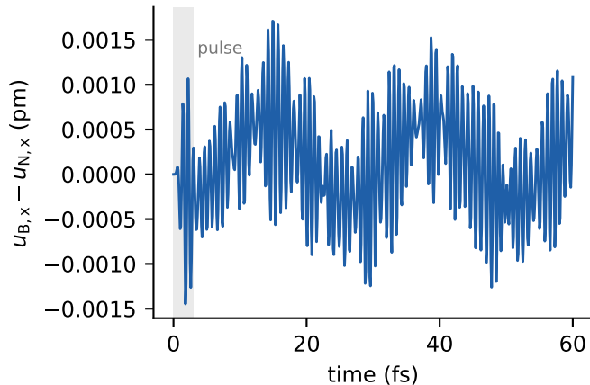
IPA, laser 5.5 eV, 10^{11} W/cm 2 , static
