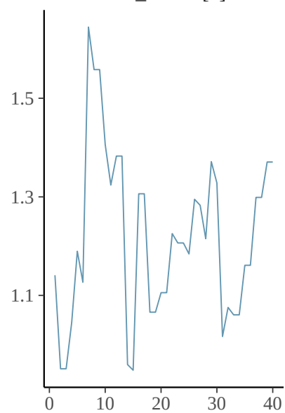
beta_denom[1]
