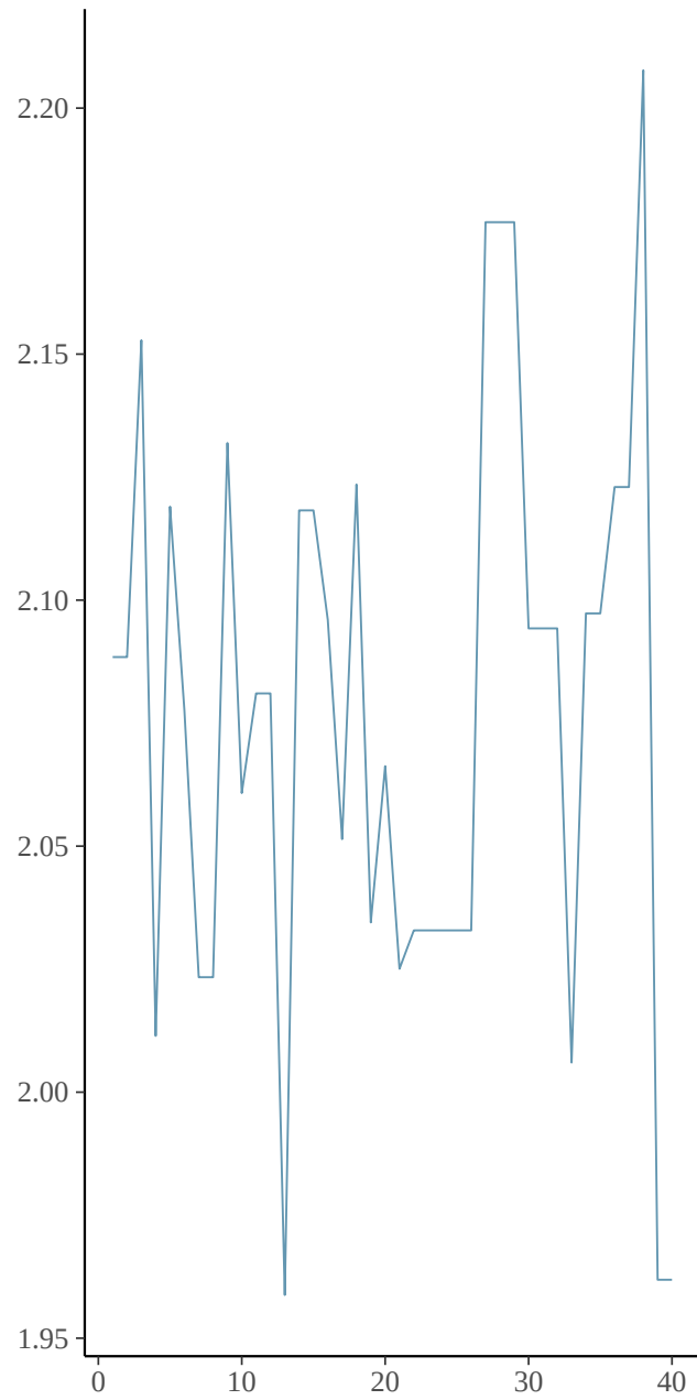
beta_num[1]
