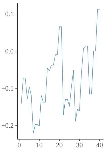
beta_denom[2]
