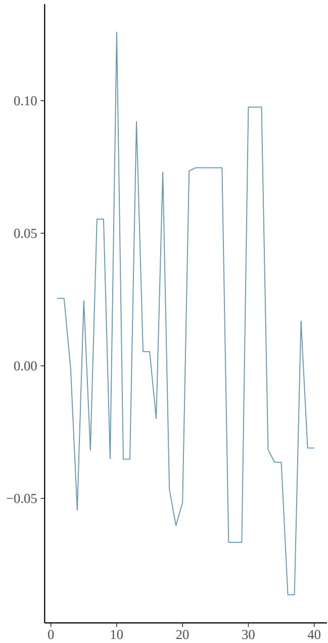
beta_num[2]
