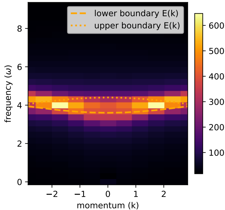
abs ED Cs(\omega, k)
