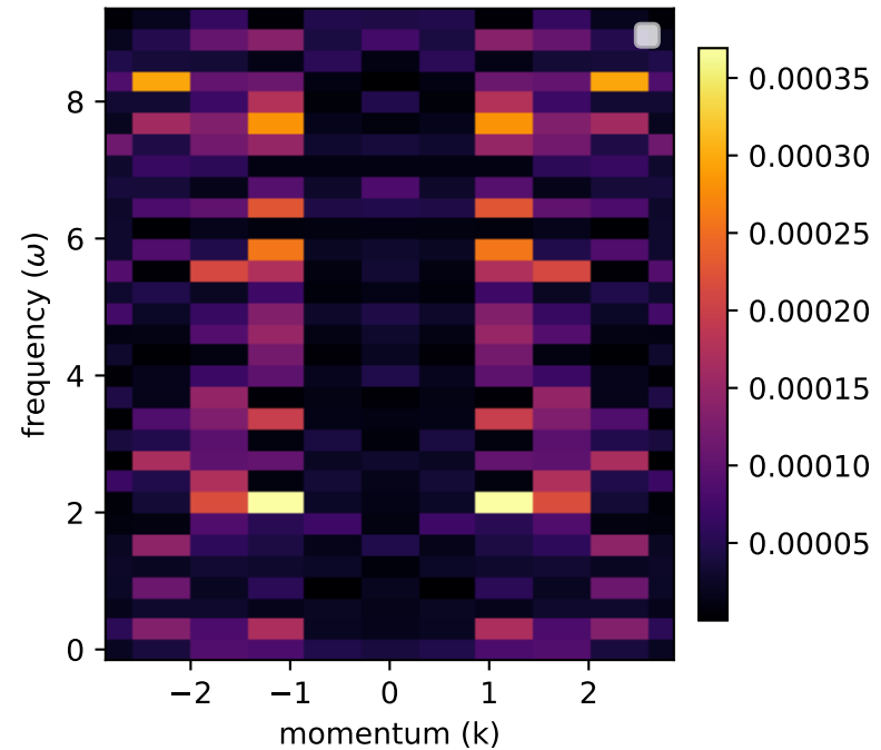
abs theo - iter
