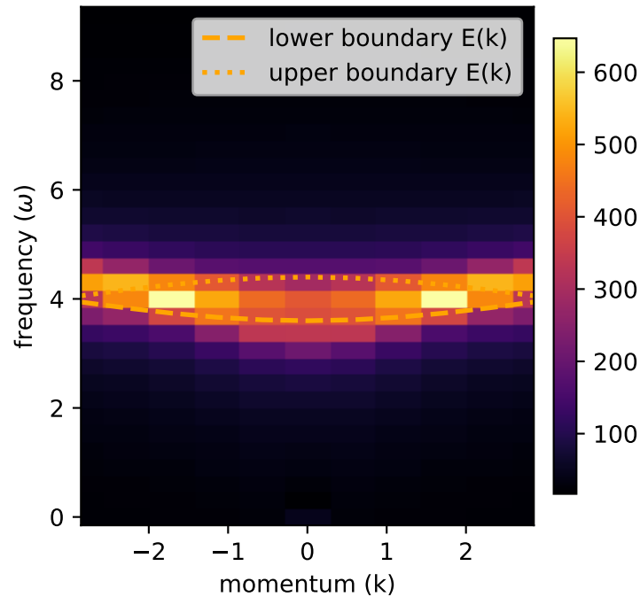
abs ID Cs(\omega, k)
