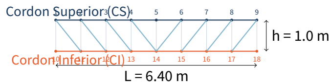
Figura 3: Cercha de transicion Warren 2D. Numeracion de nodos y miembros.
