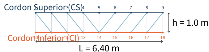
Figura 2: Cercha de transicion Warren 2D. Numeracion de nodos y miembros.
