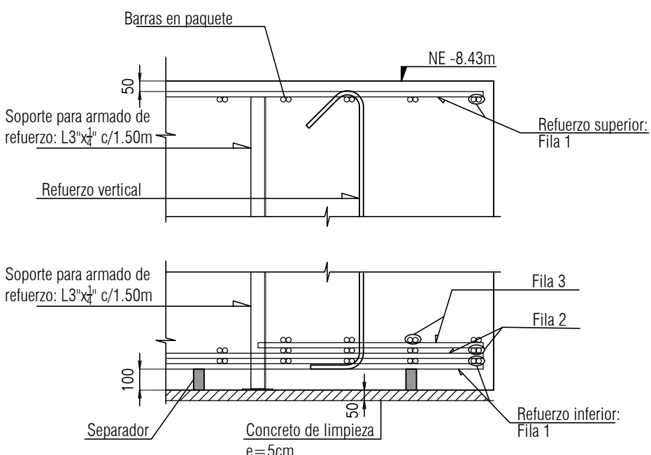
DETALLE TÍPICO ARMADO REFUERZO escala 1:25
