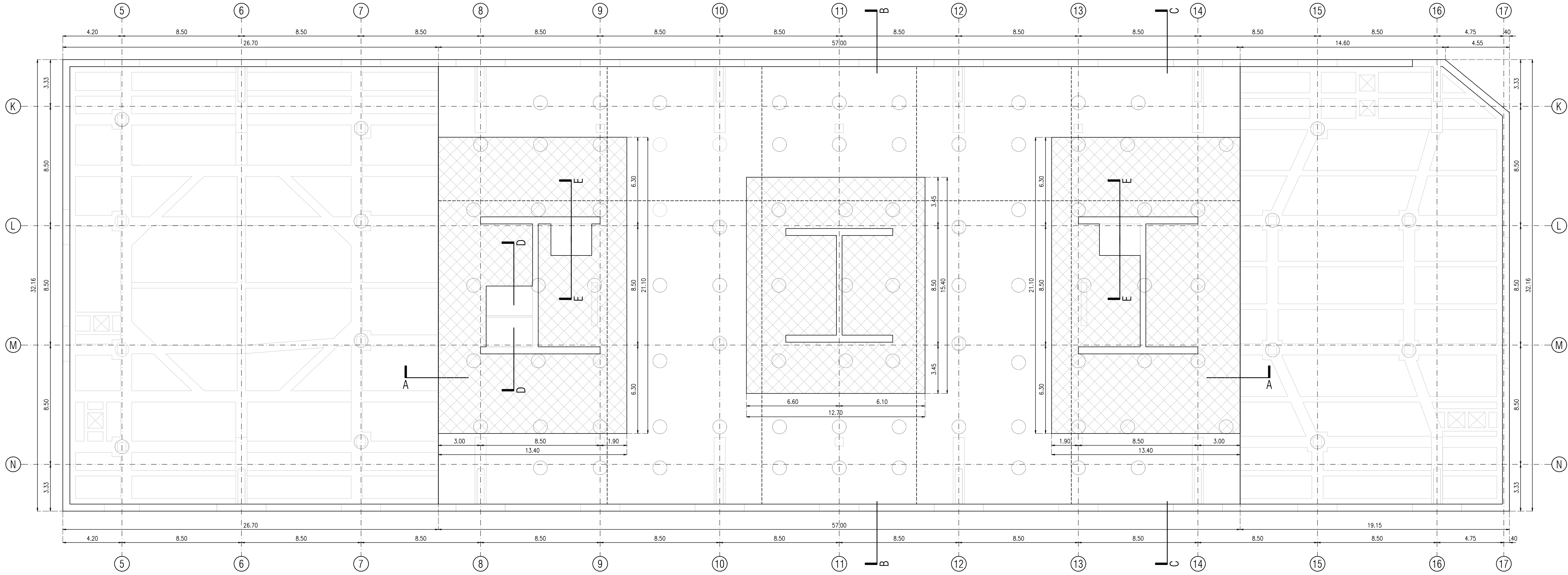
REFUERZO A CORTANTE escala 1:150
