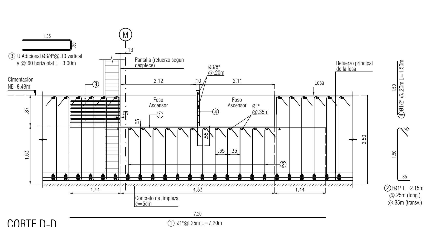
CORTE D-D escala 1:50
