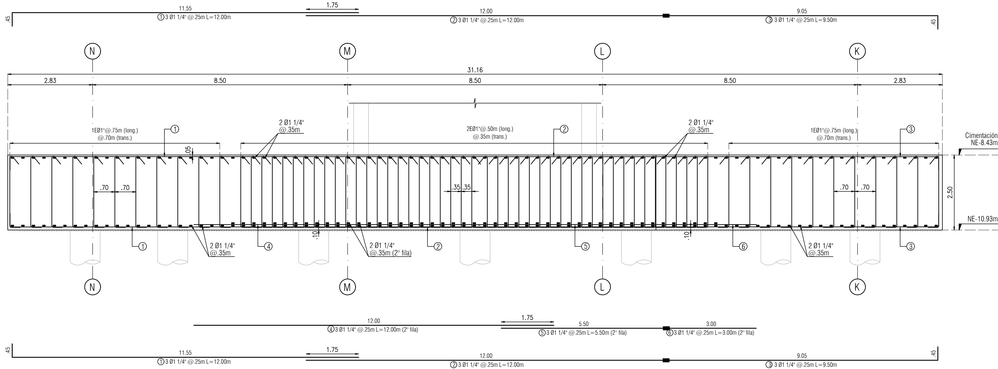
CORTE B-B escala 1:75
