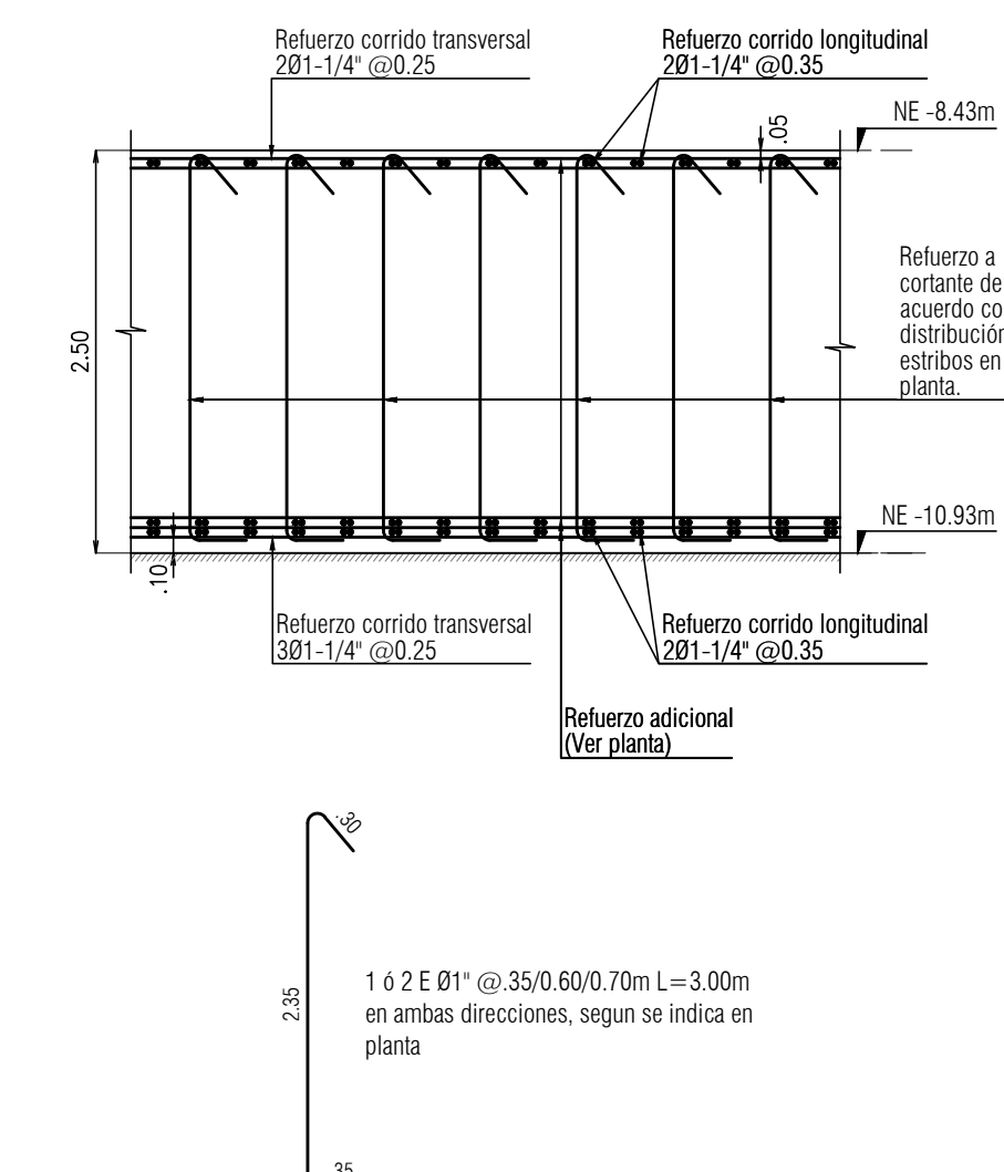
CORTE TÍPICO LOSA h=2.50m escala 1:50
