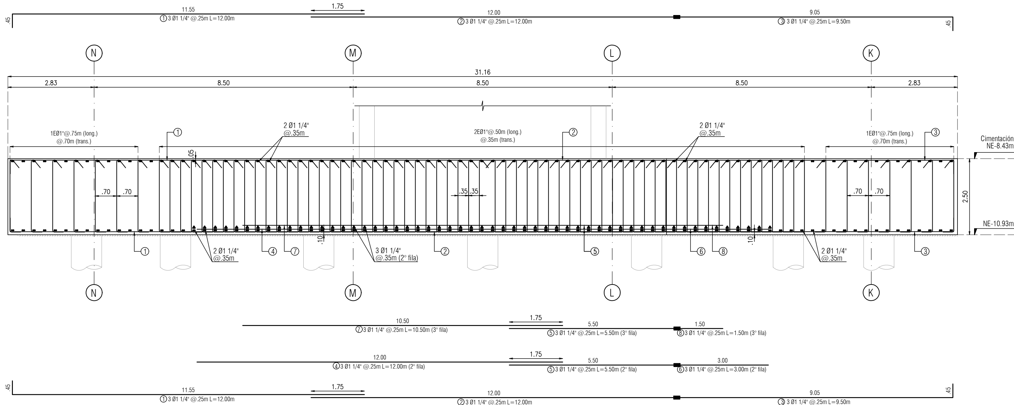
CORTE C-C escala 1:75
