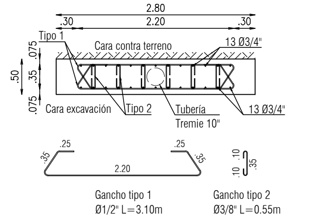
CORTE D-D - BR2 DISTRIBUCION FLEJES - T1 escala 1:50
