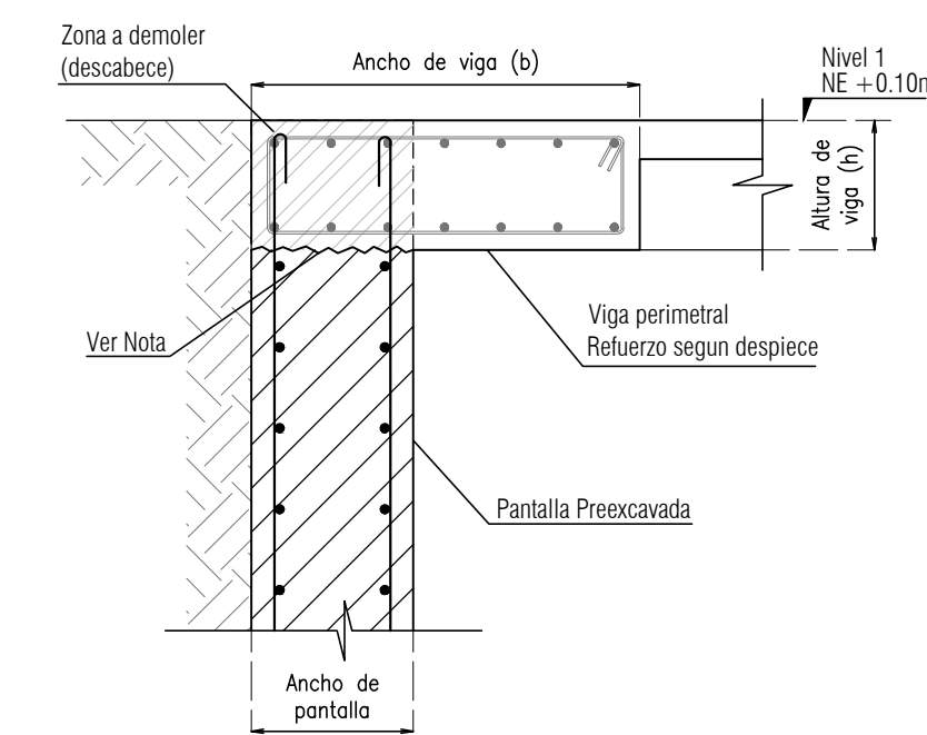
DETALLE VIGA PERIMETRAL SOBRE PANTALLA PREEXCAVADA escala 1:25
