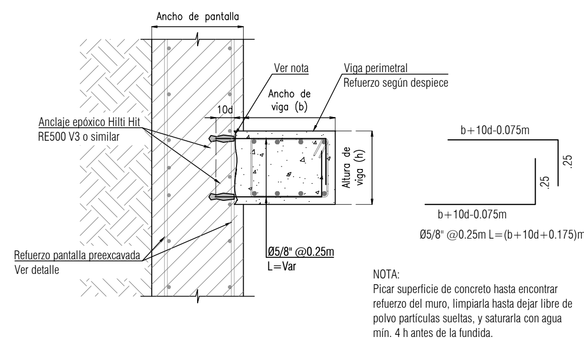
DETALLE 1 ANCLAJE VIGA PERIMETRAL A PANTALLA PREEXCAVADA Y PILOTES TANGENTES escala 1:20
