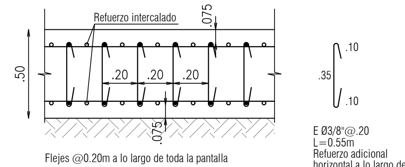
CORTE B-B REFUERZO HORIZONTAL PANTALLA PREEXCAVADA PP2 Y PP3 escala 1:20
