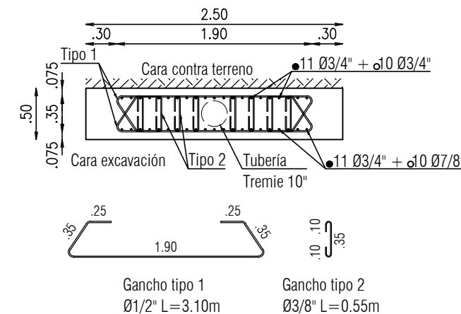
CORTE A-A - BR1 DISTRIBUCION FLEJES - T2 escala 1:50
