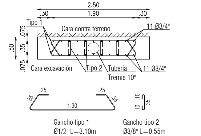
CORTE B-B - BR1 DISTRIBUCION FLEJES - T1 escala 1:50
