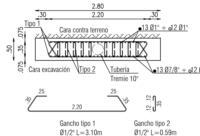
CORTE C-C - BR2 DISTRIBUCION FLEJES - T2 escala 1:50
