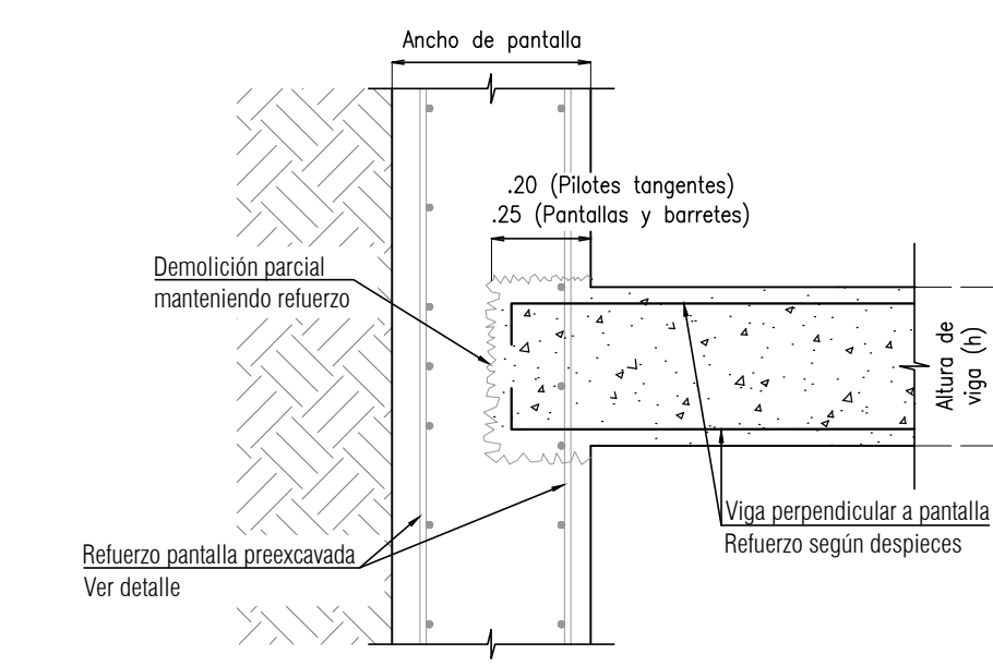
DETALLE 2 ANCLAJE DE VIGAS PERPENDICULARES A PANTALLA PREEXCAVADA Y PILOTES TANGENTES escala 1:20
