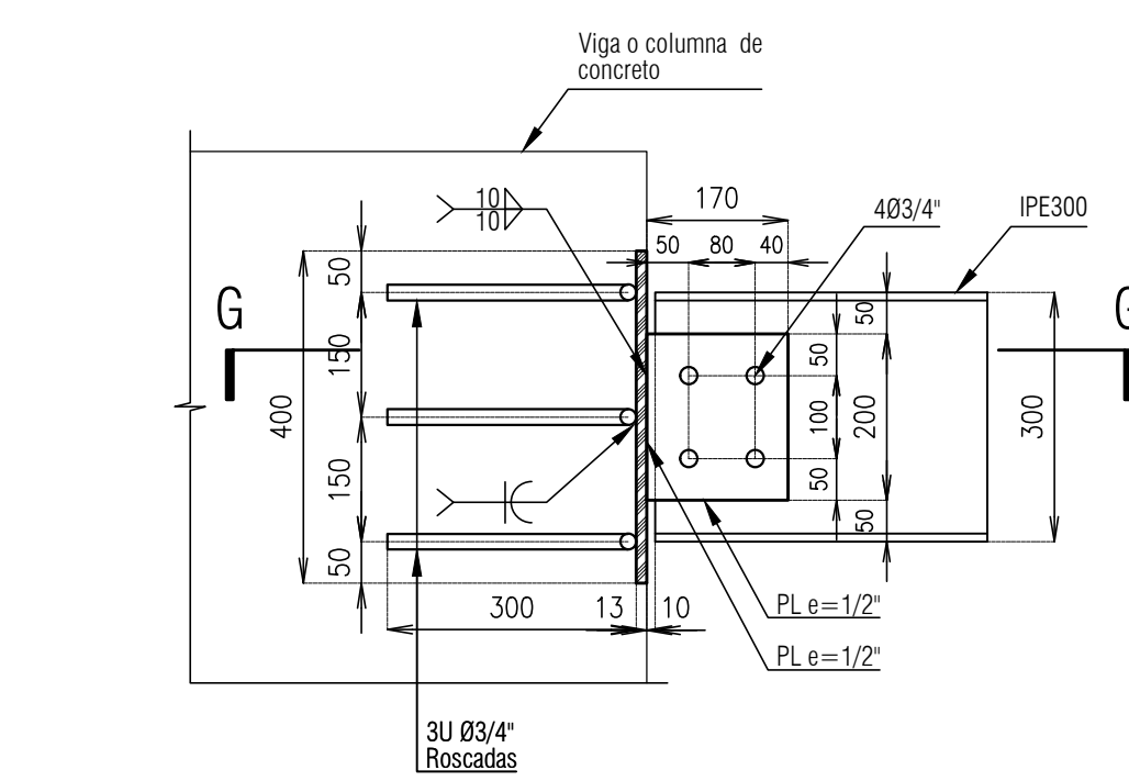
Conexión IPE300 a Concreto (Niveles 8 a 23) escala 1:10
