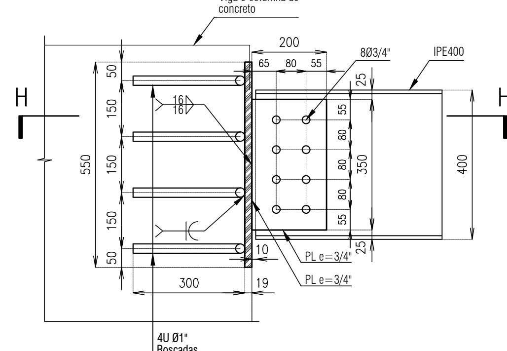
Conexión IPE400 a Concreto (Terraza) escala 1:10
