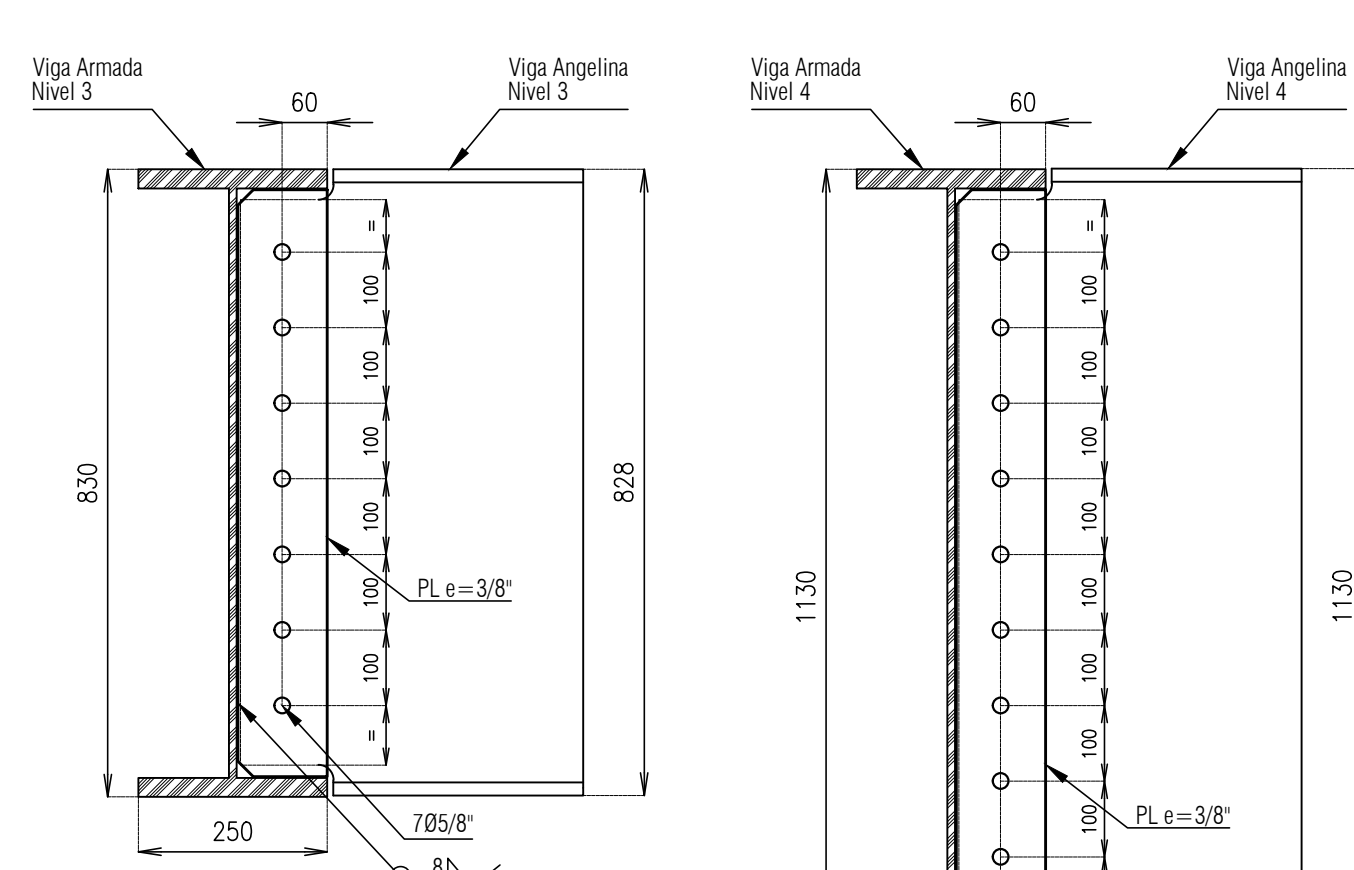
Conexiones de Vigas Angelinas a Vigas Armadas escala 1:10
