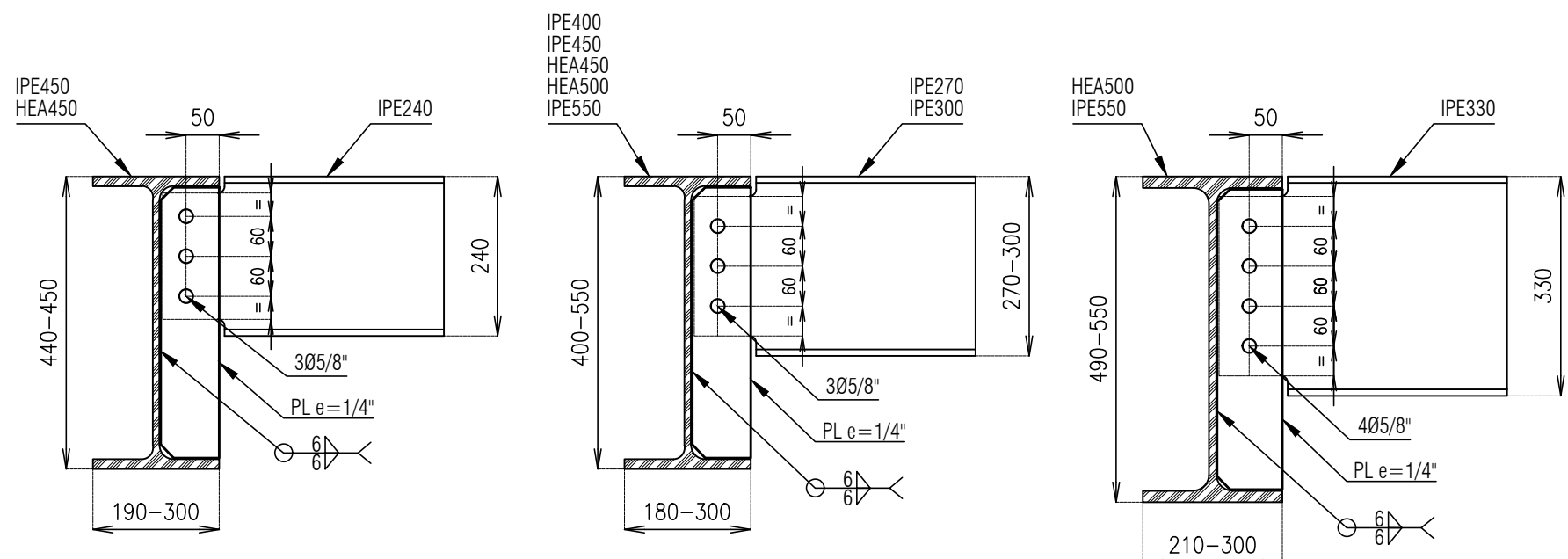
Conexiones típicas de Viguetas escala 1:10
