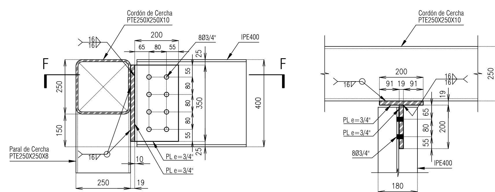
Conexión IPE400 a Cercha de Fachada Niveles 8 a 23 escala 1:10
