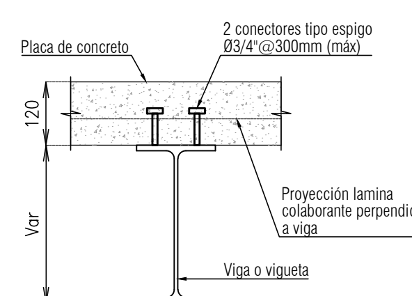
Detalle conectores de cortante escala 1:10
