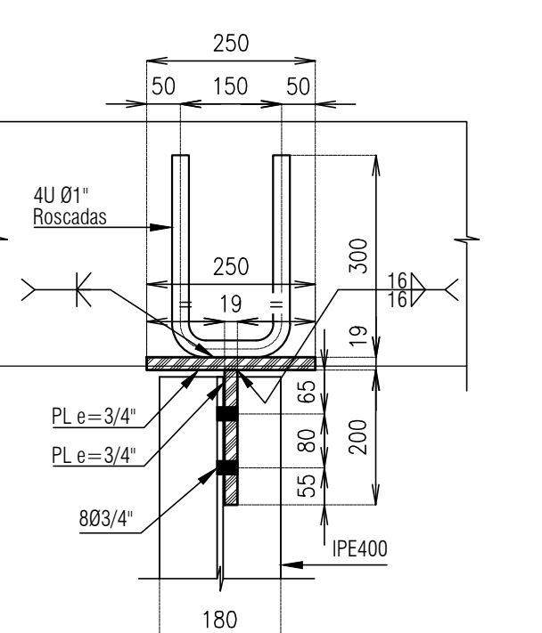
Sección H-H escala 1:10
