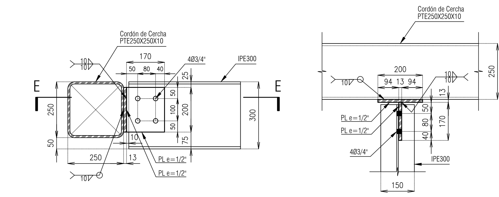
Conexión IPE300 a Cercha de Fachada Niveles 8 a 23 escala 1:10
