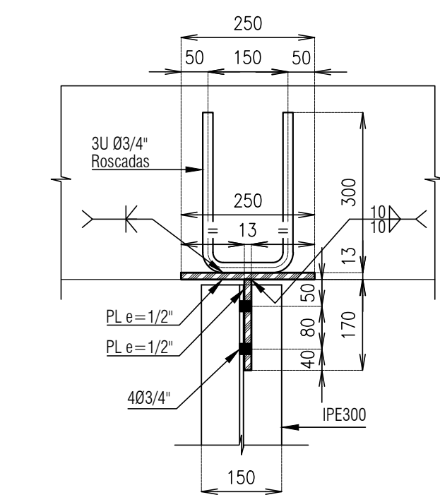
Sección G-G escala 1:10
