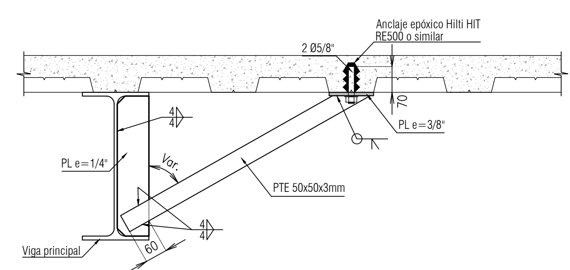
Detalles típicos de arriostamiento de vigas escala 1:10
