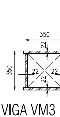
VIGA VM3 escala 1:20
