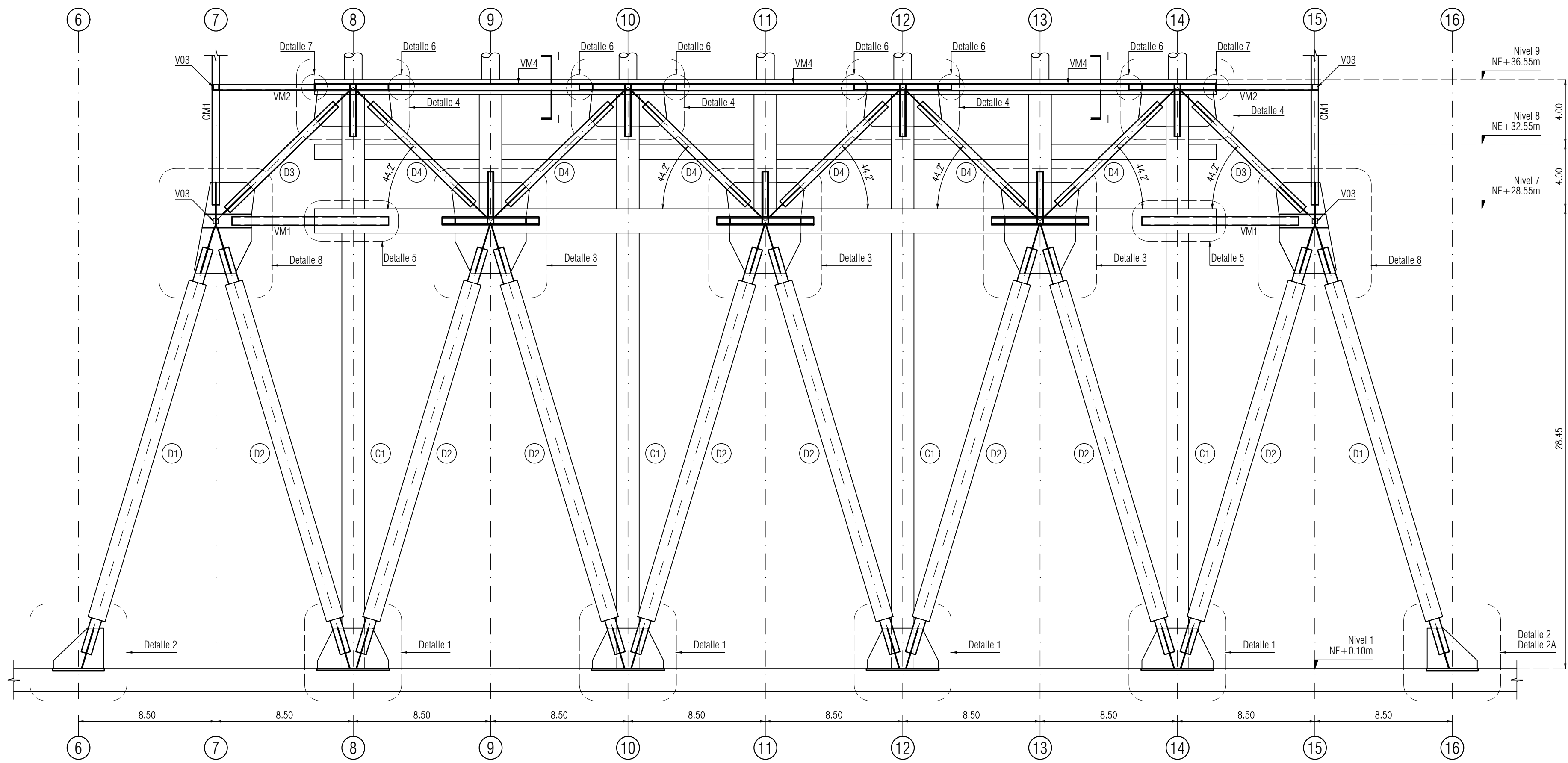
ALZADO DIAGONALES NIVEL 1 A 9 escala 1:100
