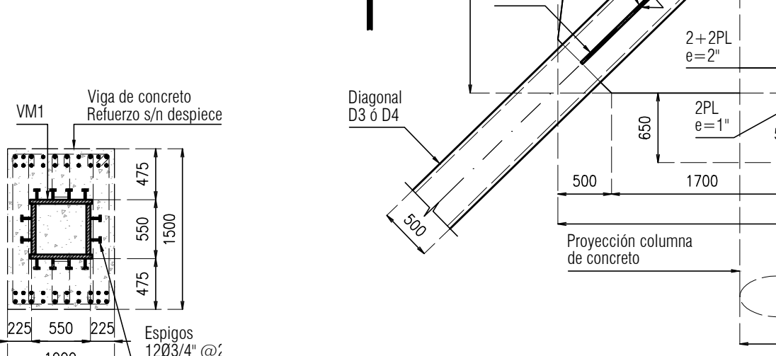
Detalle 4 escala 1:50
