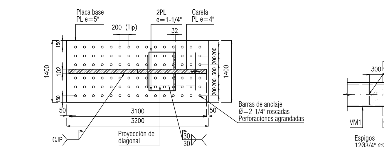
Corte C-C escala 1:50
