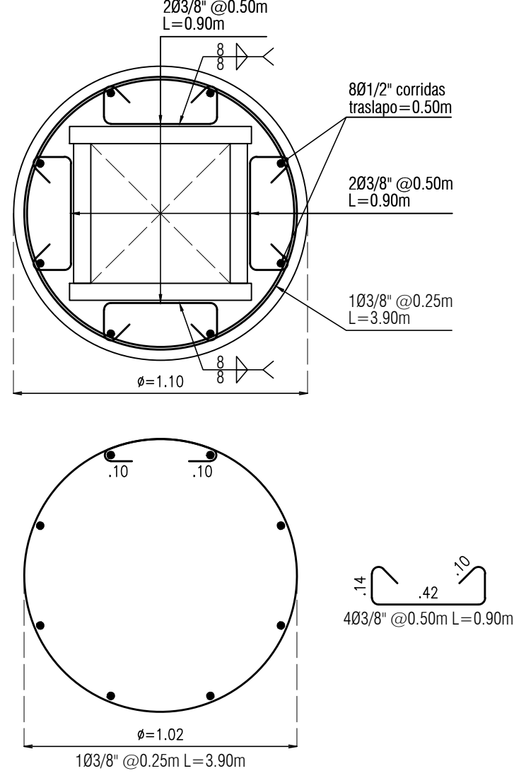
REFUERZO CAMISA DIAGONALES D1 Y D2 escala 1:20
