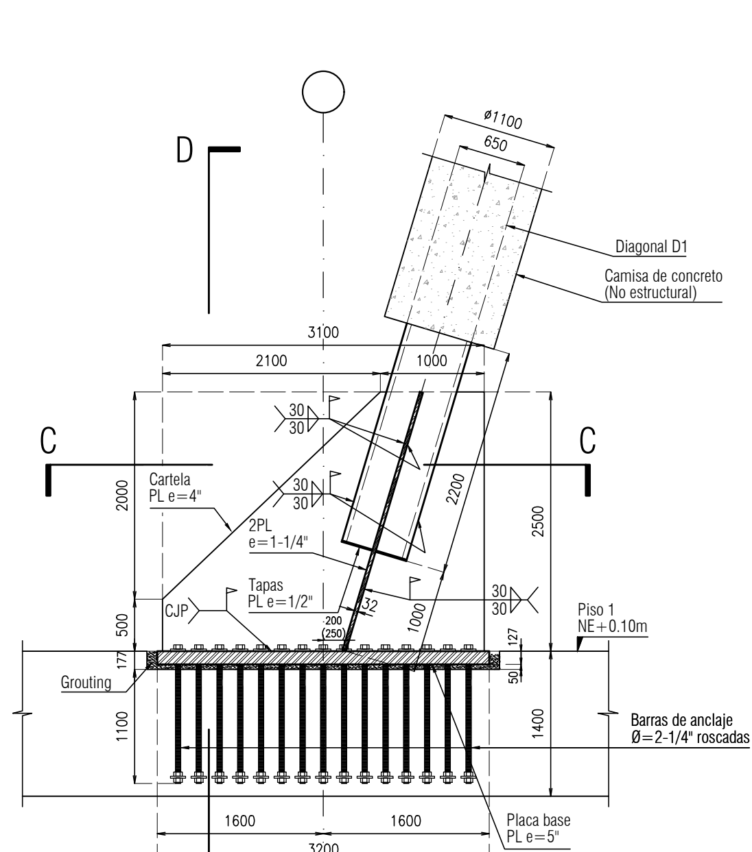
Detalle 2 escala 1:50
