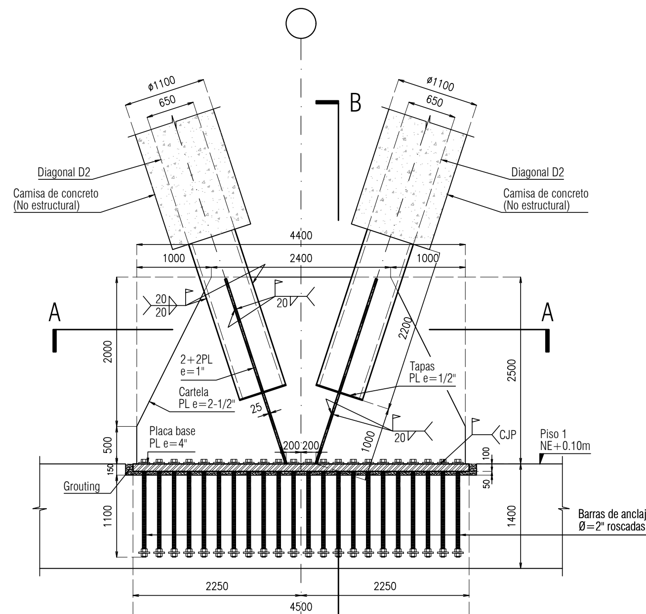
Detalle 1 escala 1:50
