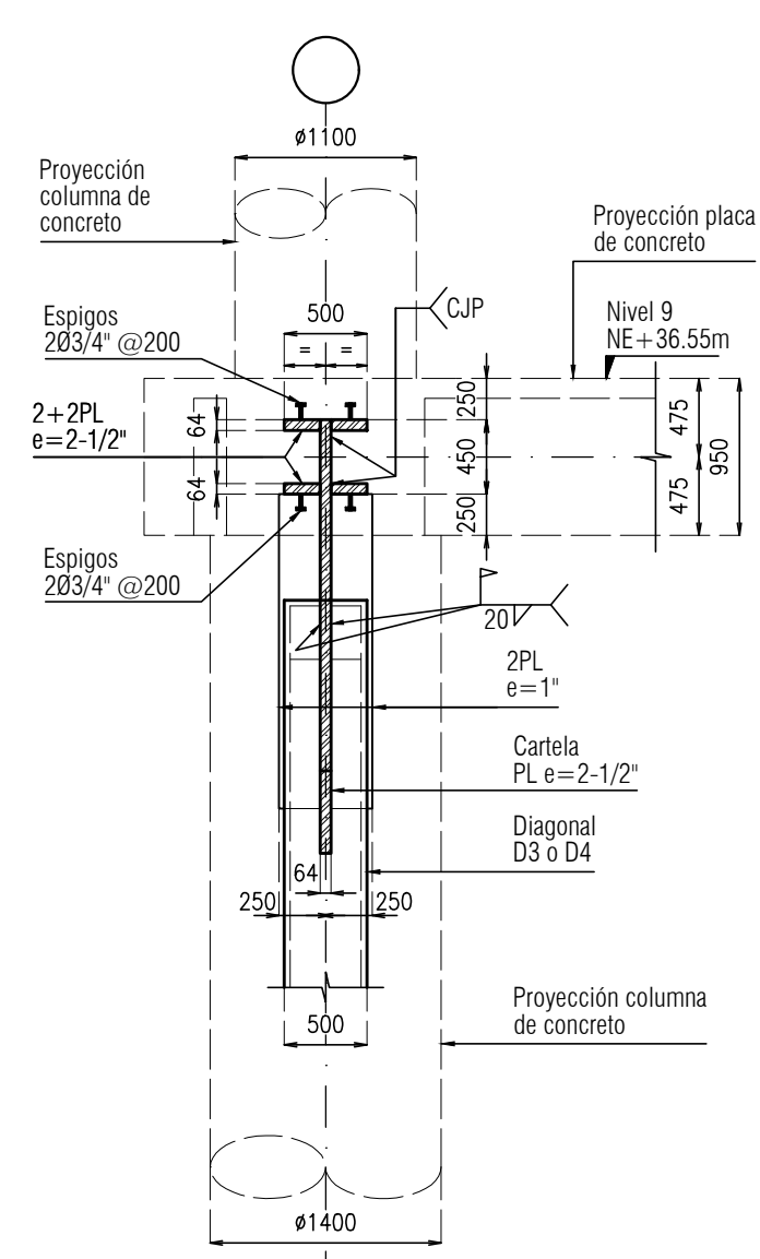
Corte G-G escala 1:50
