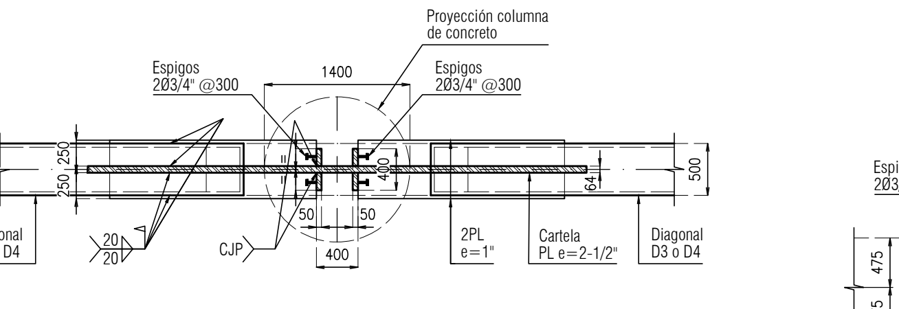
Corte F-F escala 1:50
