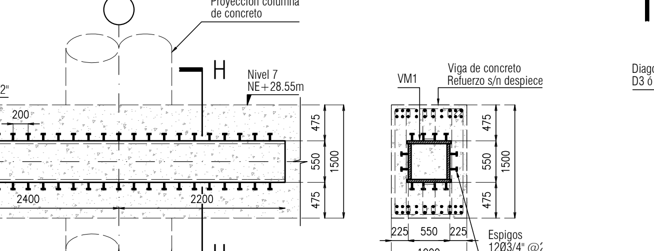
Detalle 5 escala 1:50
