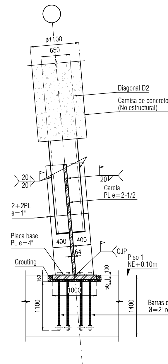
Corte B-B escala 1:50
