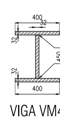
VIGA VM4 escala 1:20
