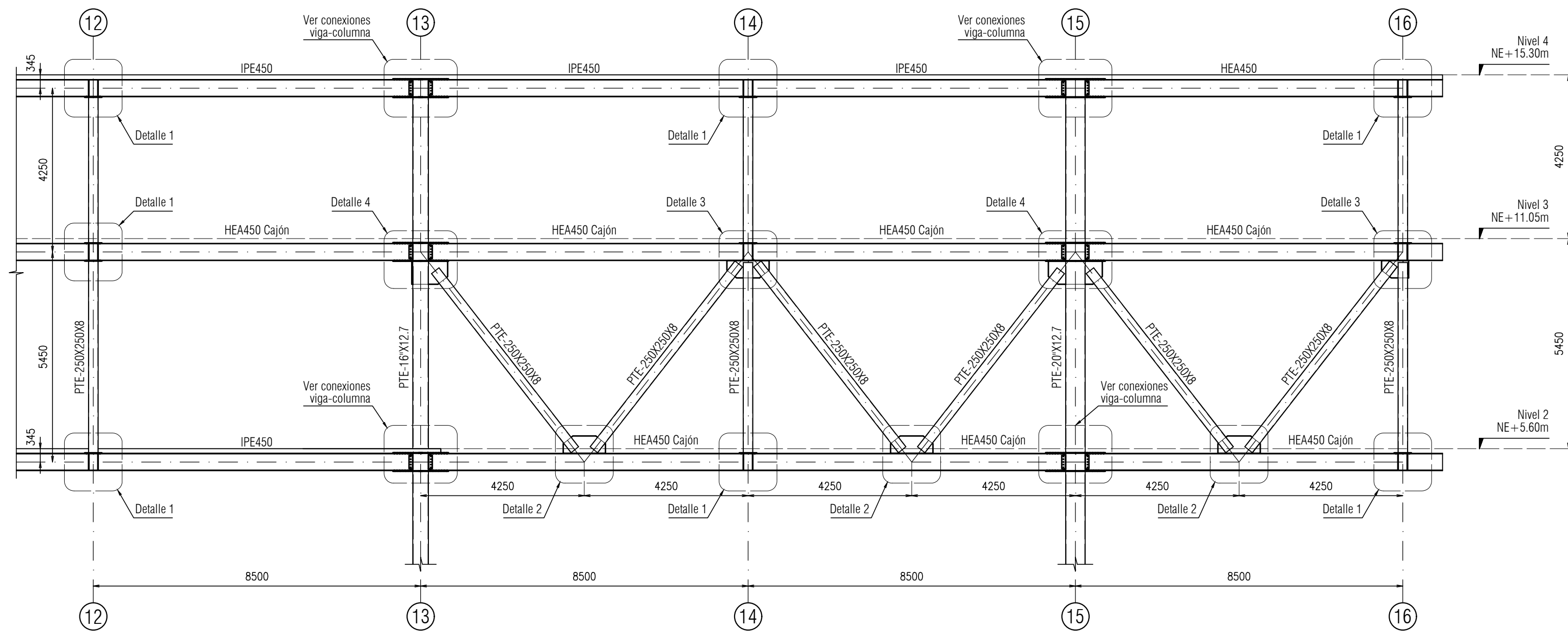
ALZADO FACHADA EJE N escala 1:100
