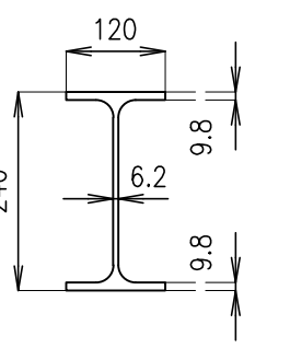
Sección IPE240 escala 1:10
