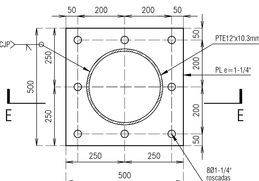
Placa Base Tensor PTE 12\"/>
