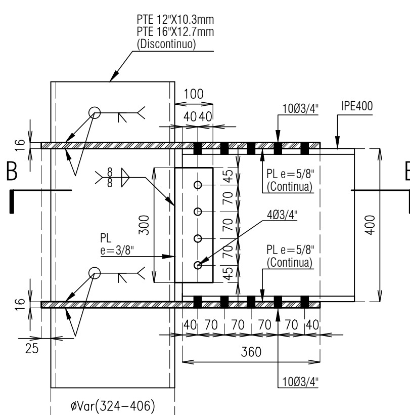
Conexión IPE400 a Columna escala 1:10
