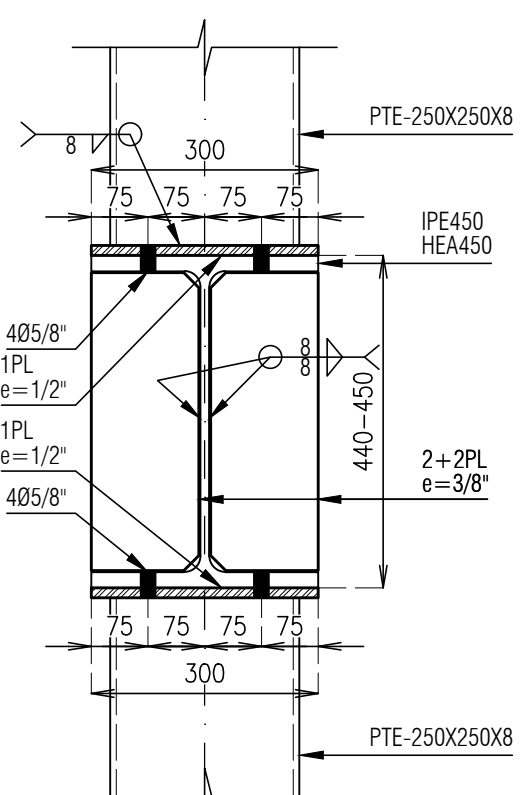
Corte A-A escala 1:10
