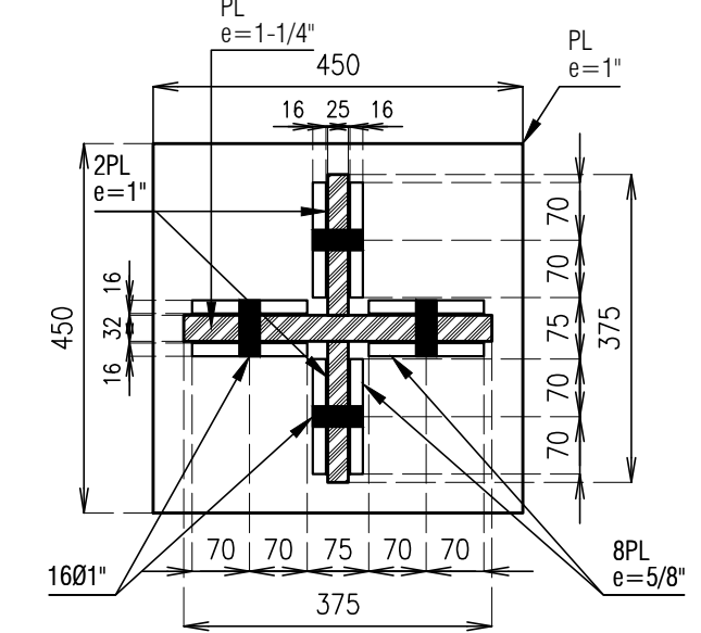
Sección G-G escala 1:10
