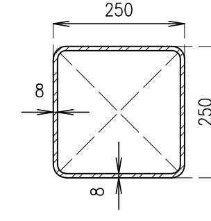
PTE-250X250X8 escala 1:10
