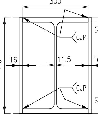
HEA450 Cajón escala 1:10
