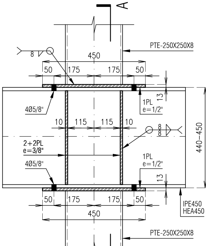
Detalle 1 escala 1:10
