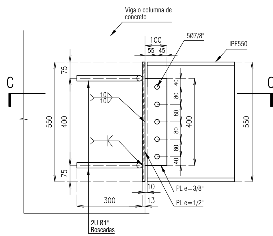
Conexión IPE550 a Concreto (N5 a N7) escala 1:10
