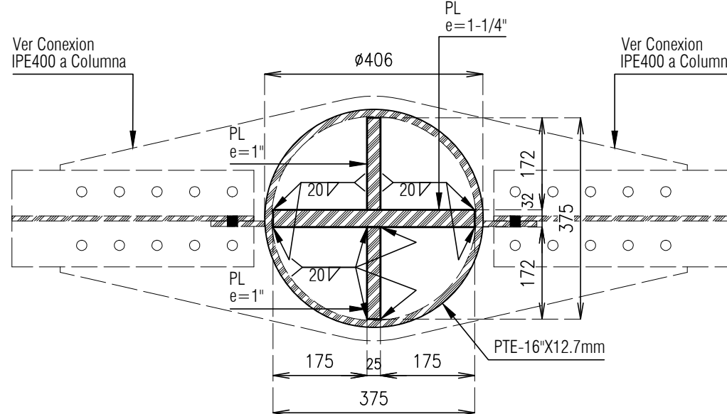
Sección F-F escala 1:10
