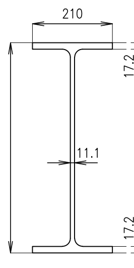
Sección IPE550 escala 1:10
