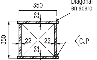
SECCION VIGA VM3 escala 1:20
