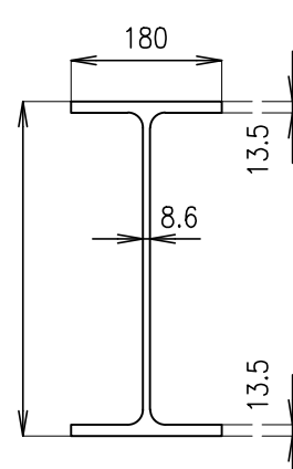
Sección IPE400 escala 1:10
