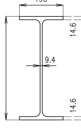
Sección IPE450 escala 1:10
