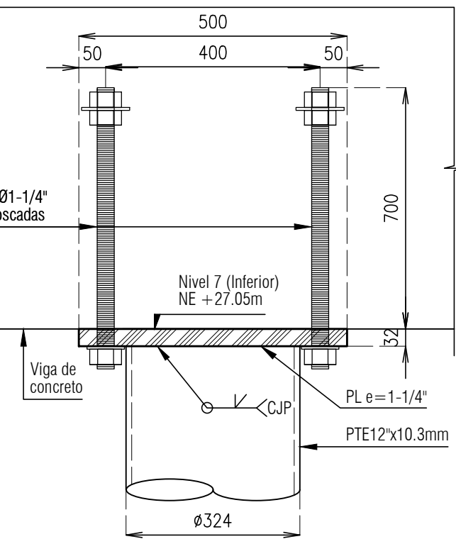
Sección E-E escala 1:10
