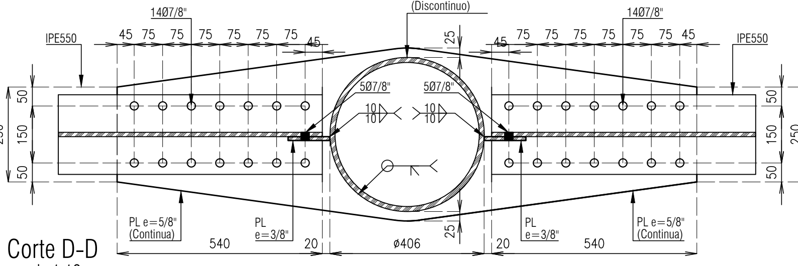
Corte D-D escala 1:10
