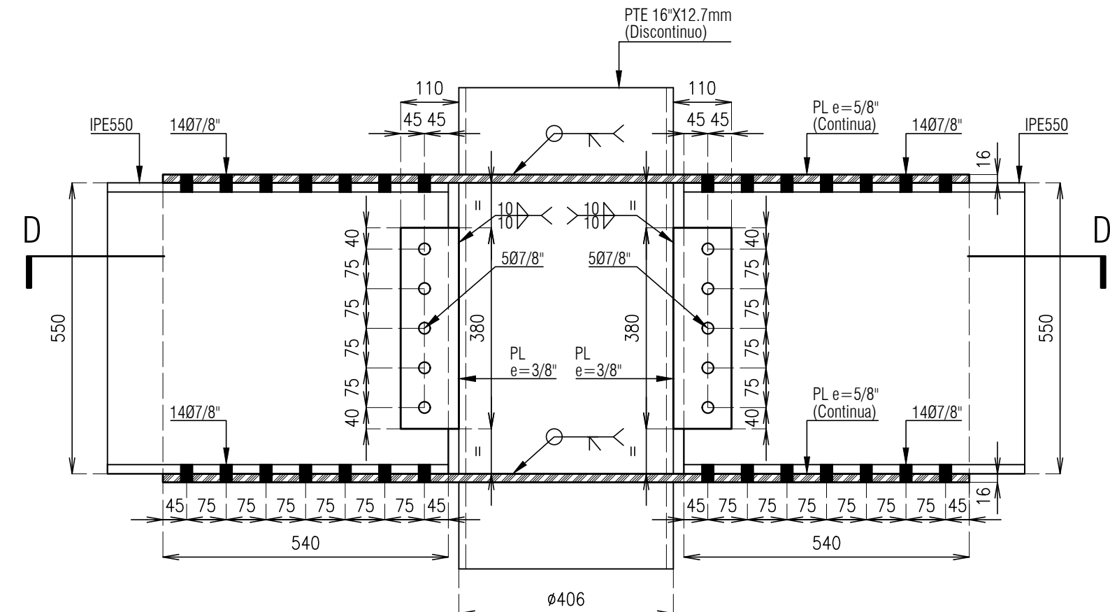
Conexión IPE550 a Columna escala 1:10
