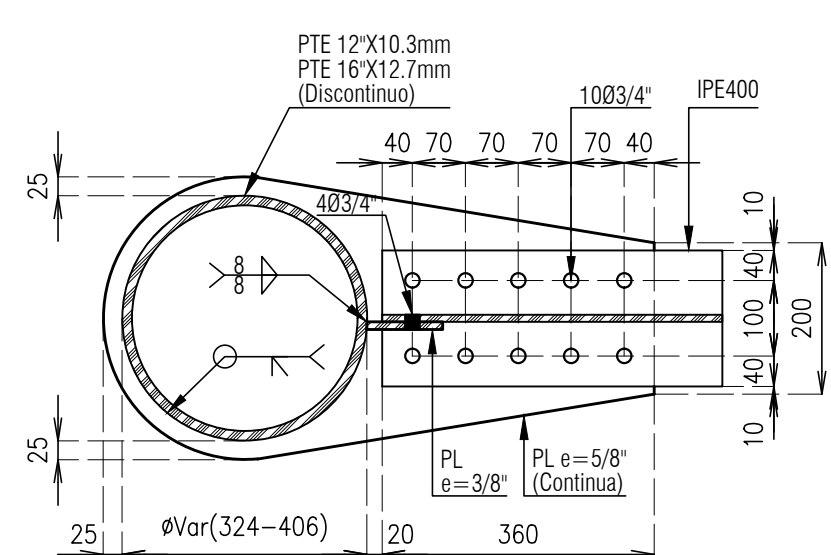
Corte B-B escala 1:10
