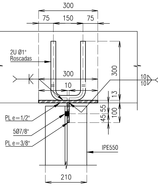
Sección C-C escala 1:10
