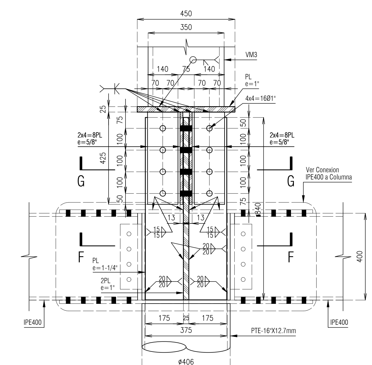
Conexión VM3 a Tensor PTE-16\"/>
