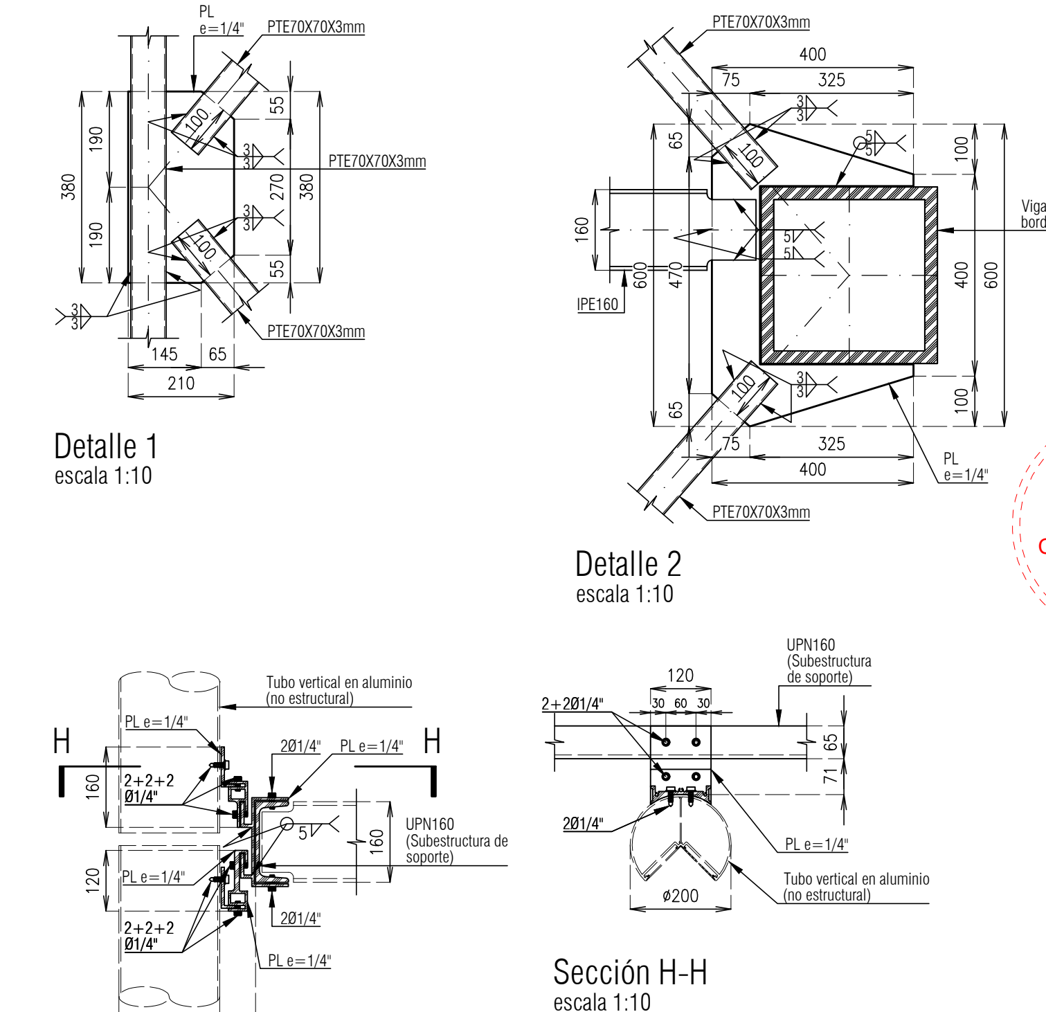
Conexión típica de tubos de aluminio de fachadas escala 1:10
