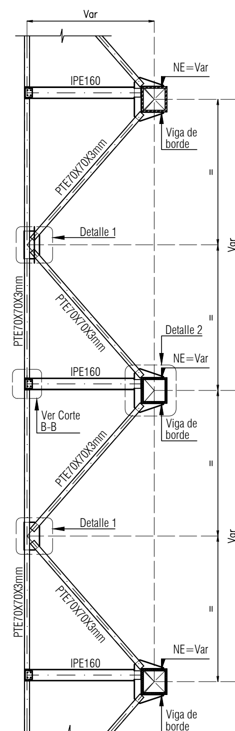
Corte D-D escala 1:50
