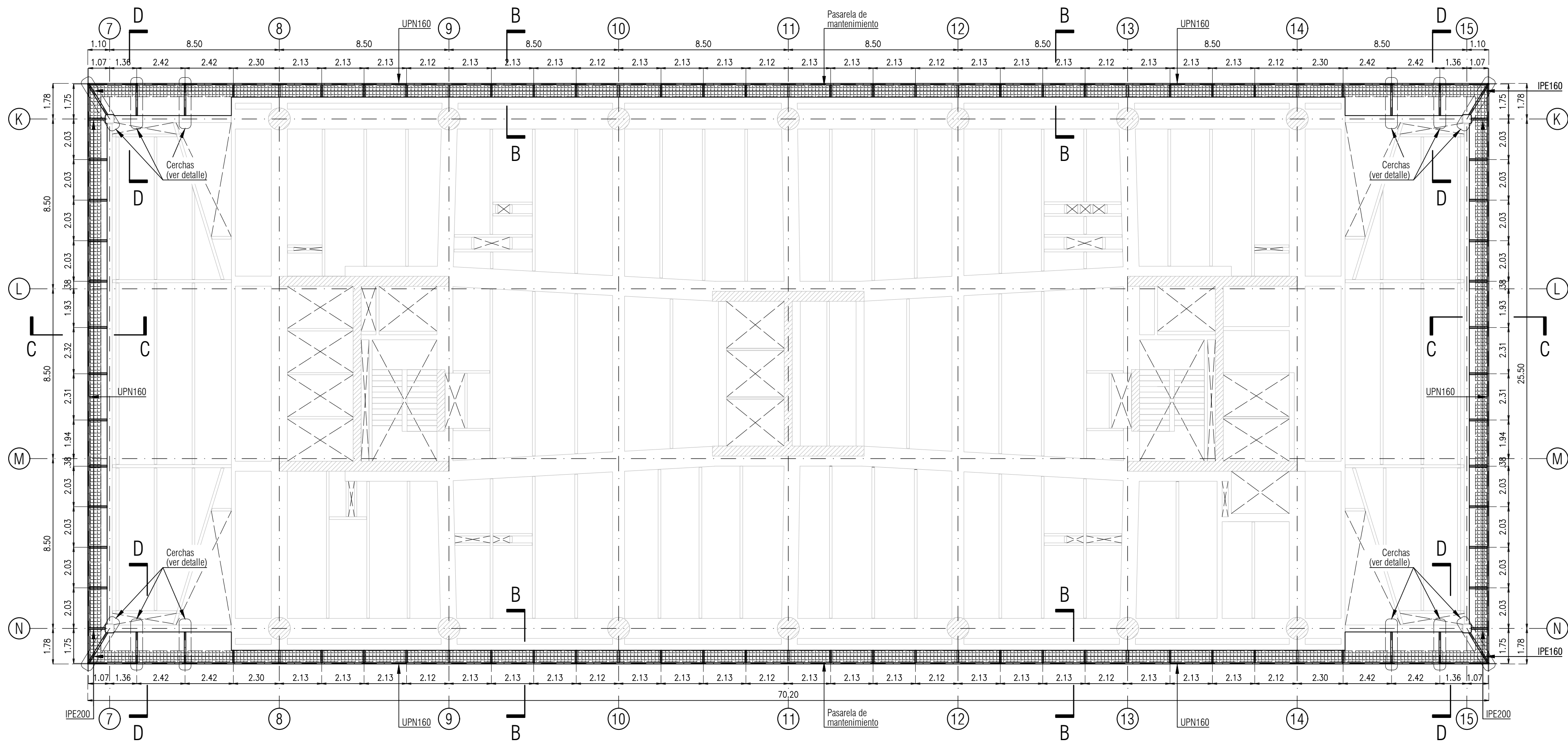
Subestructura de Fachada Niveles 7 a Terraza escala 1:150
