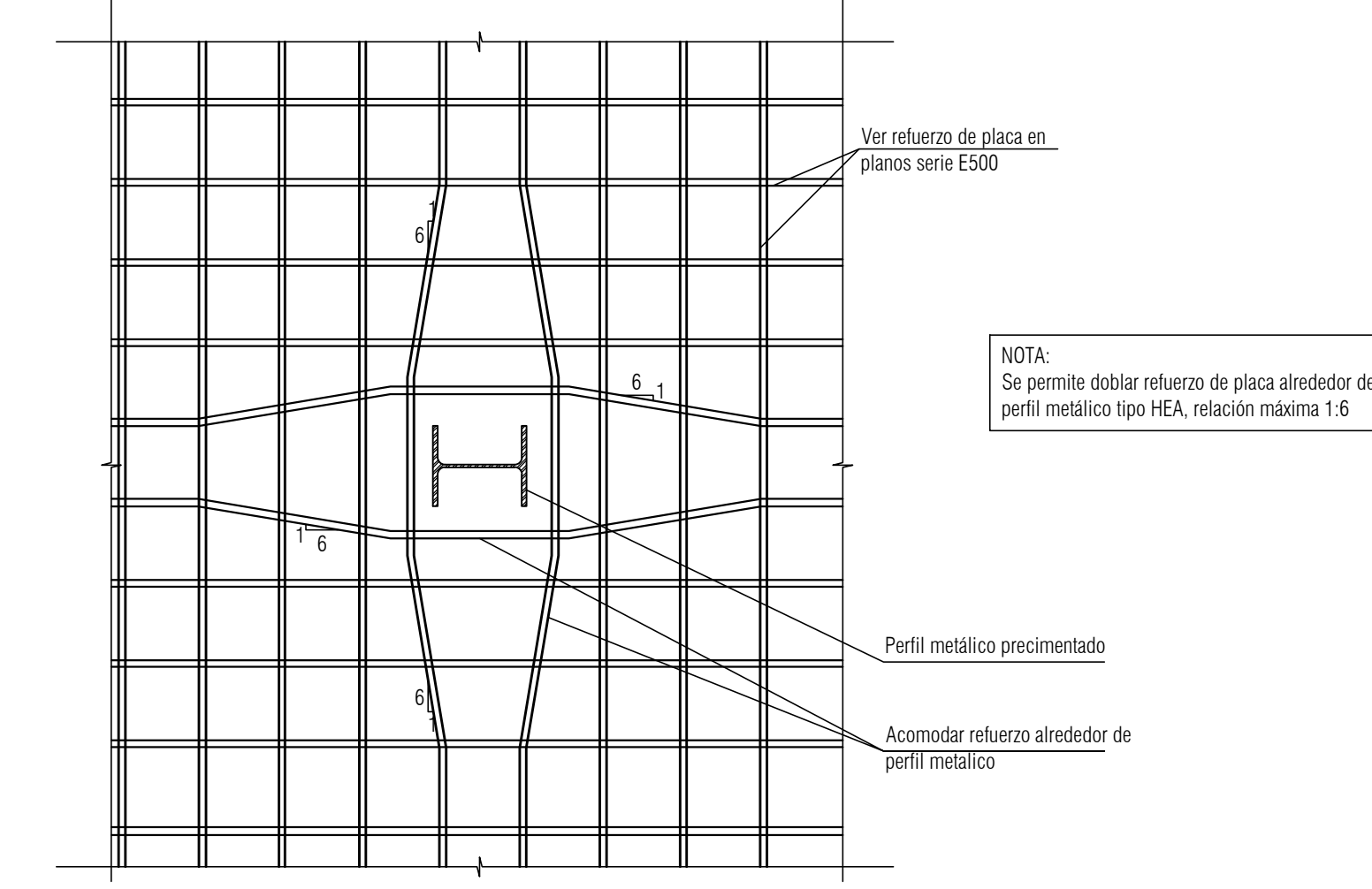
DETALLE ARMADO DE REFUERZO DE PLACA DE SUBPRESIÓN SOBRE PERFIL METÁLICO TIPO HEA escala 1:25
