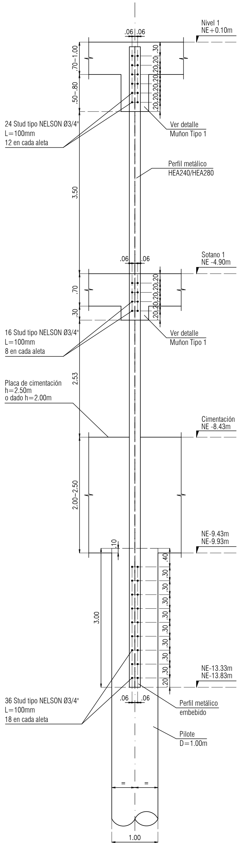
DETALLES TÍPICOS DE PERFILES HEA EMBEBIDOS PARA APOYO TEMPORAL DE PLACAS ANDEN escala 1:50
