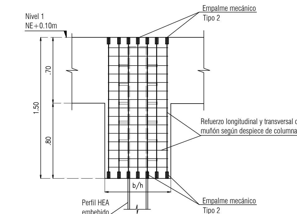
DETALLE MUÑÓN TIPO 1 escala 1:25
