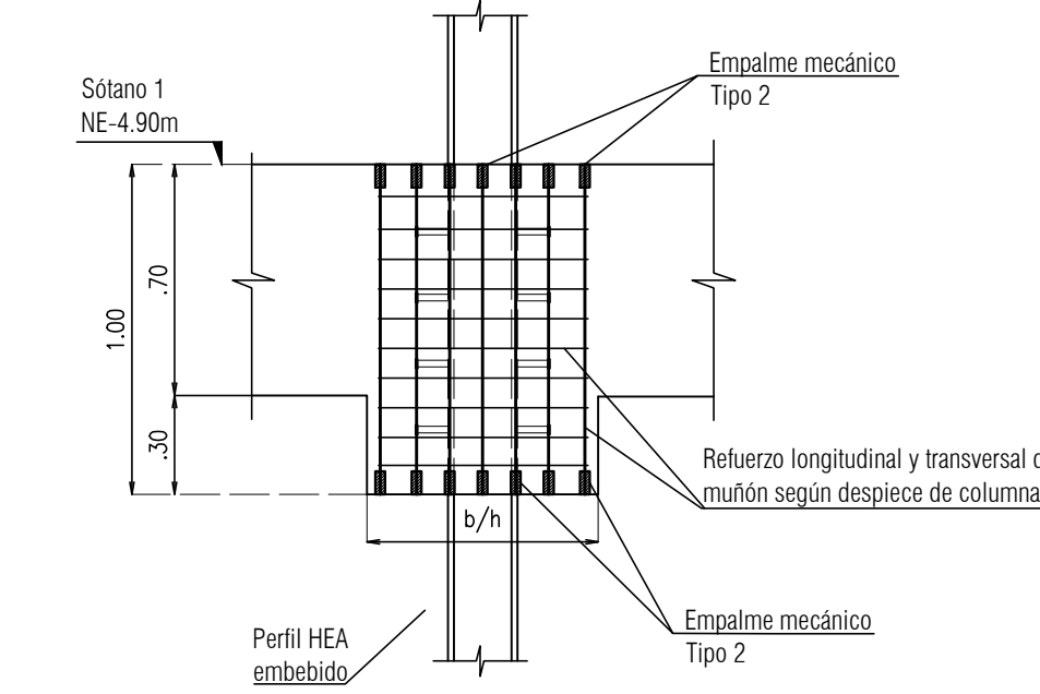
REFUERZO MUÑÓN TIPO 2 escala 1:25
