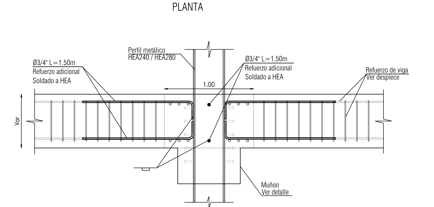
NOTA: - Máxima inclinación para el doblado en planta de las barras de refuerzo: 1:6
