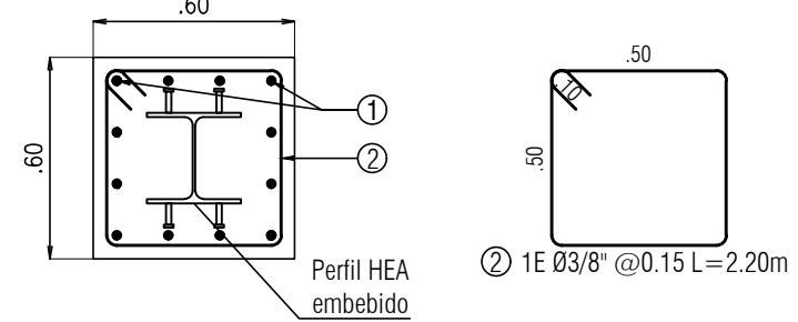
CORTE A-A escala 1:25
