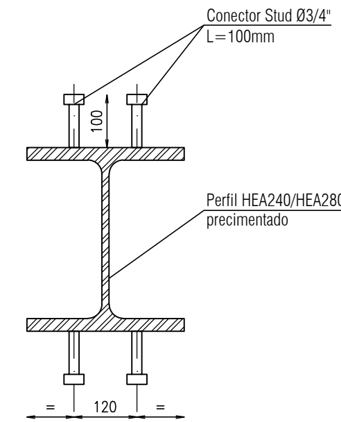
DETALLE CONECTORES A PERFIL HEA escala 1:10
