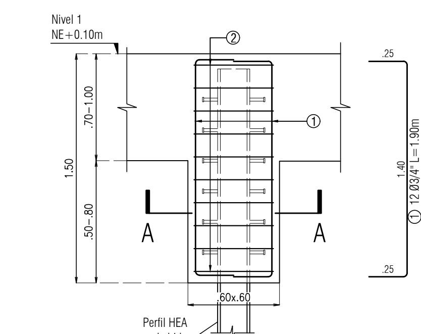
DETALLE MUÑÓN TIPO 3 escala 1:25
