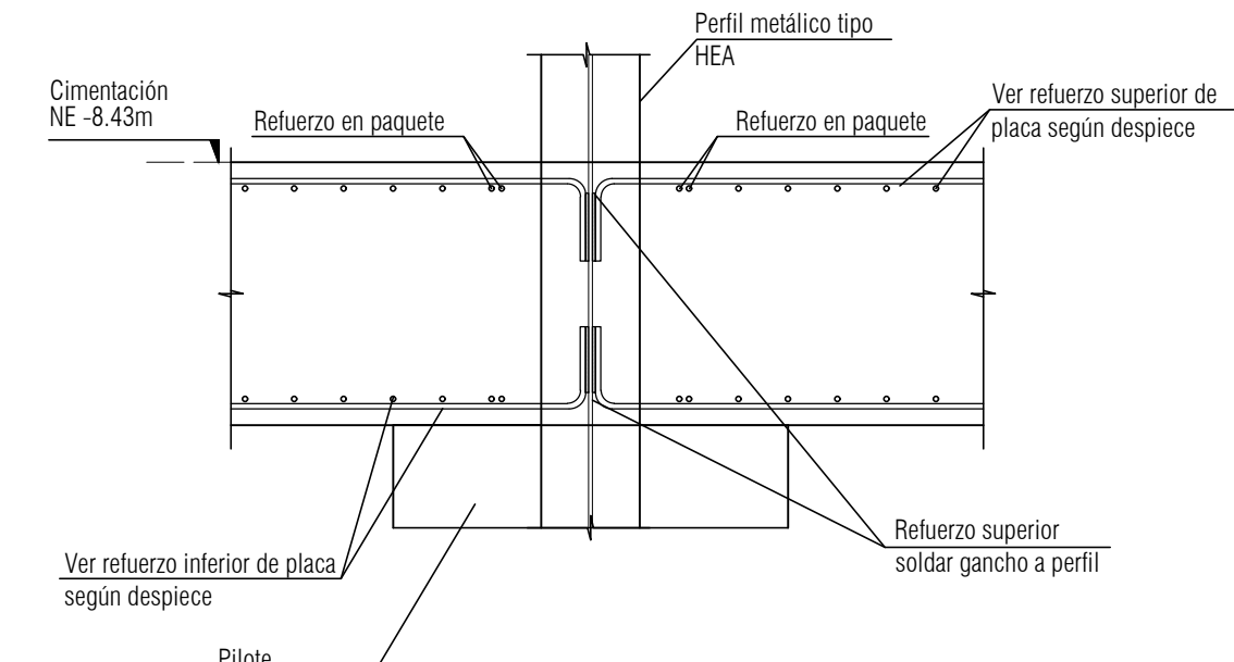
DETALLE ARMADO DE REFUERZO DE PLACA DE SUPRESIÓN SOBRE PERFIL METÁLICO TIPO HEA (ALTERNATIVA) escala 1:25
