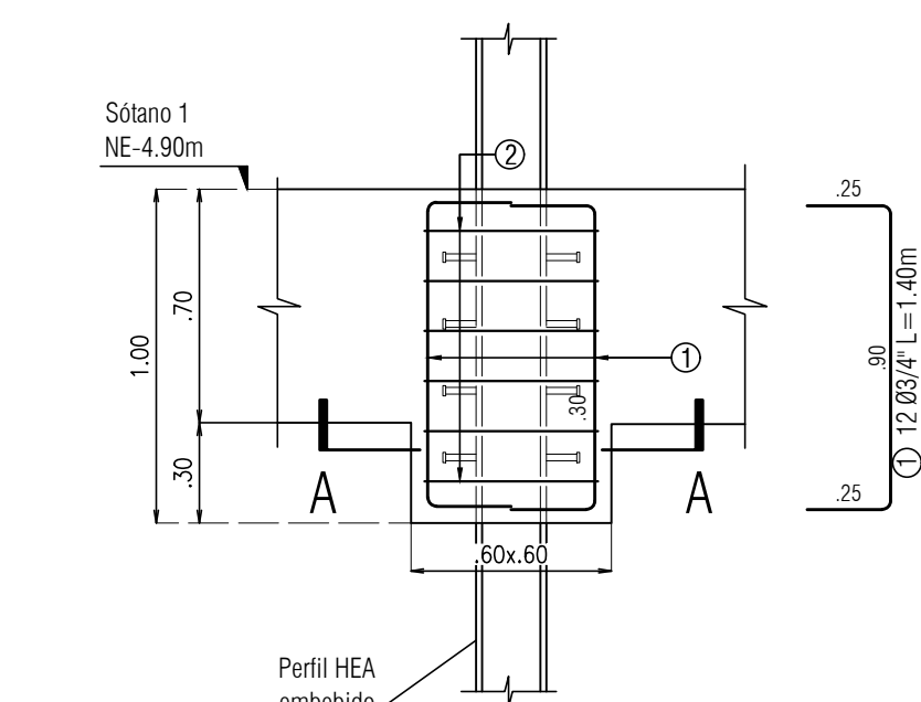
REFUERZO MUÑÓN TIPO 4 escala 1:25
