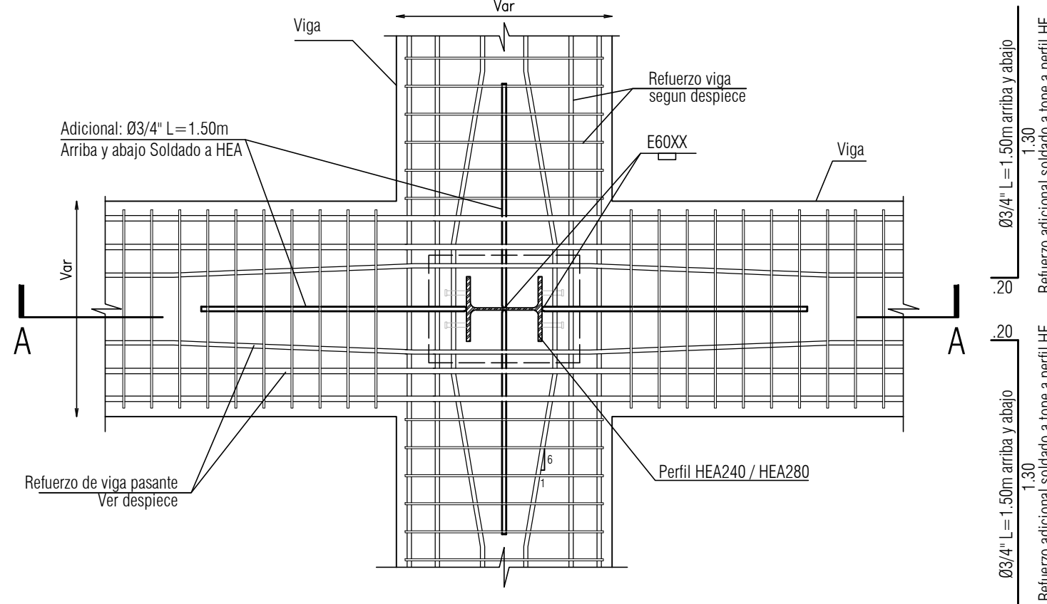
NOTA: - Máxima inclinación para el doblado en planta de las barras de refuerzo: 1:6
