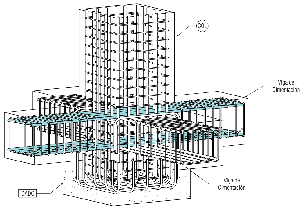
AXONOMETRÍA escala
