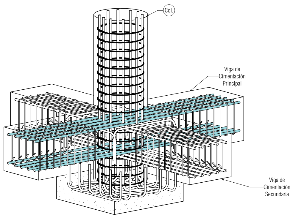
AXONOMETRÍA escala
