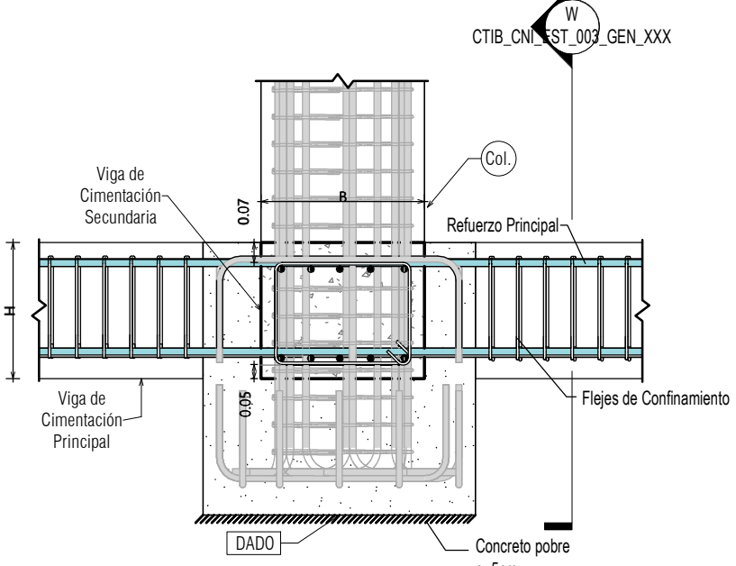
CORTE X-X
