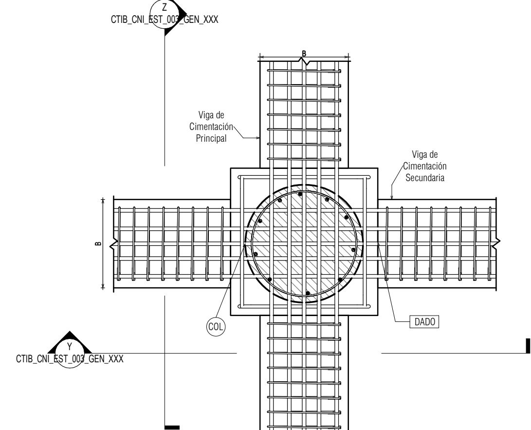
PLANTA
