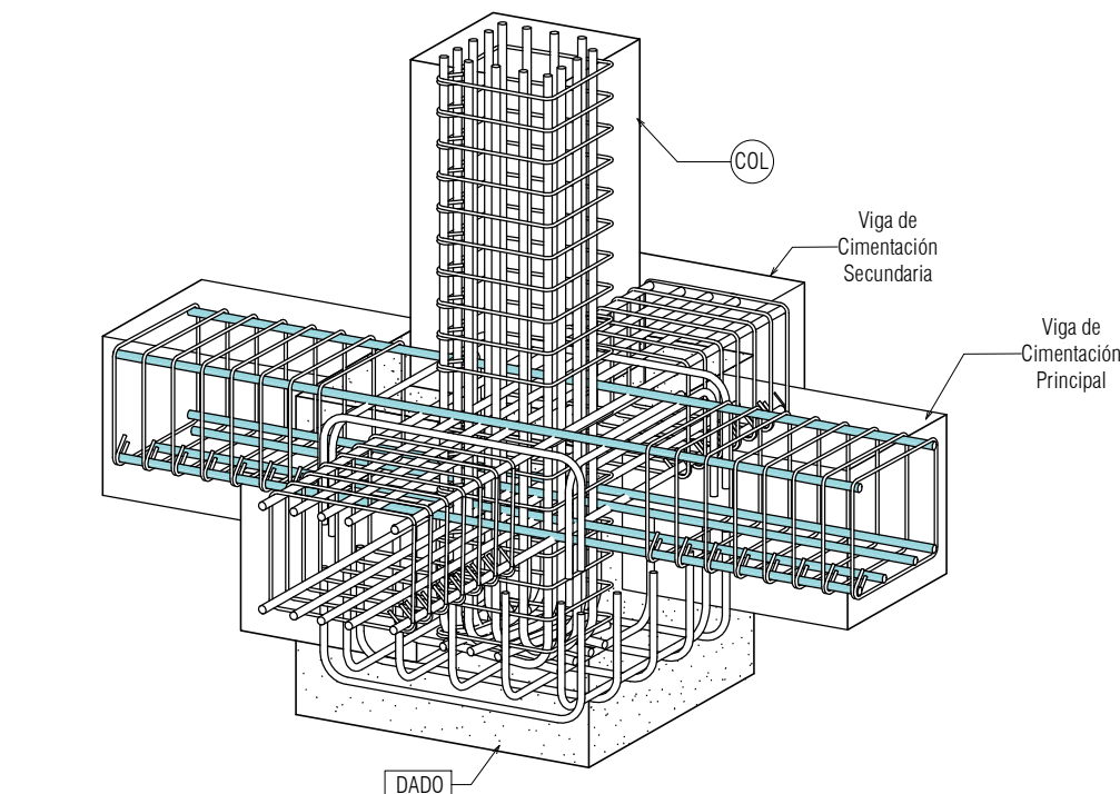
AXONOMETRÍA escala
