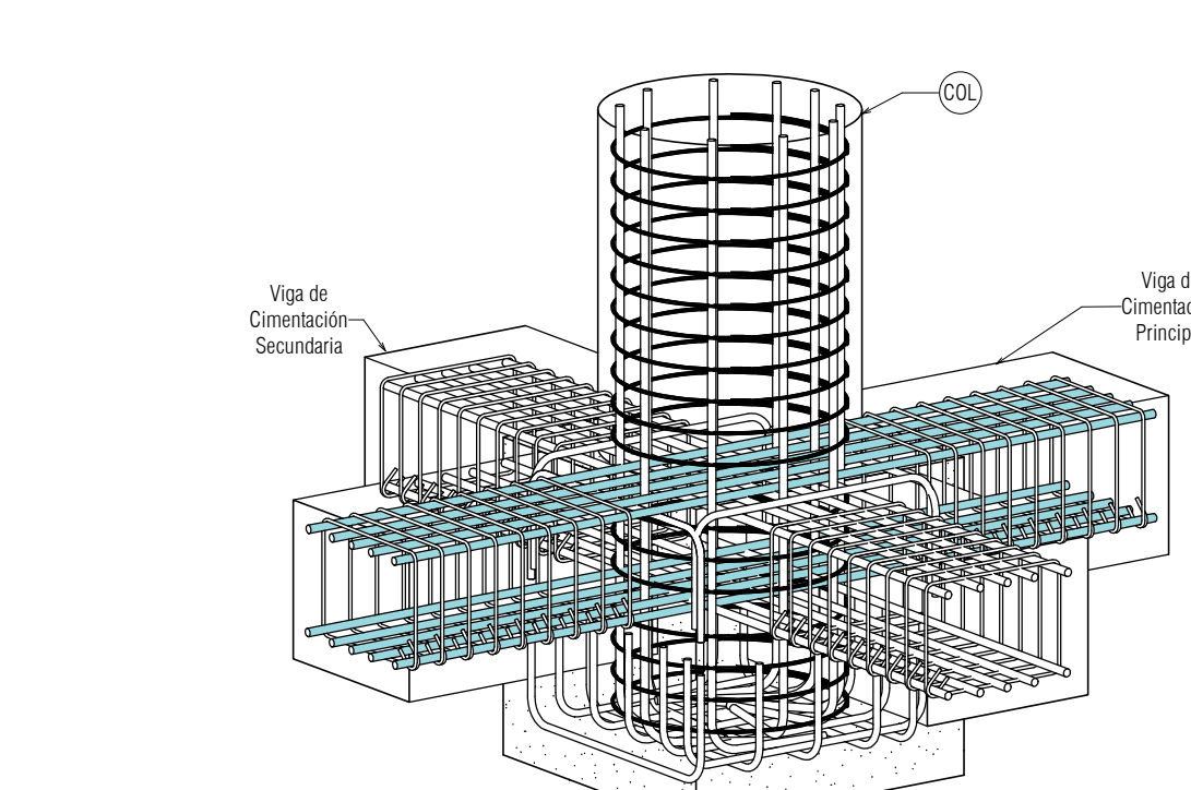
AXONOMETRÍA escala
