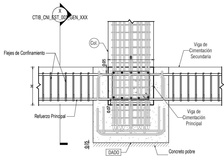
CORTE W-W
