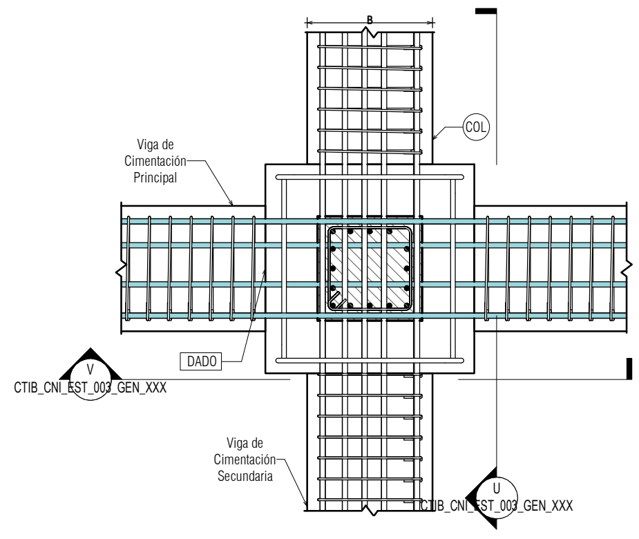
PLANTA
