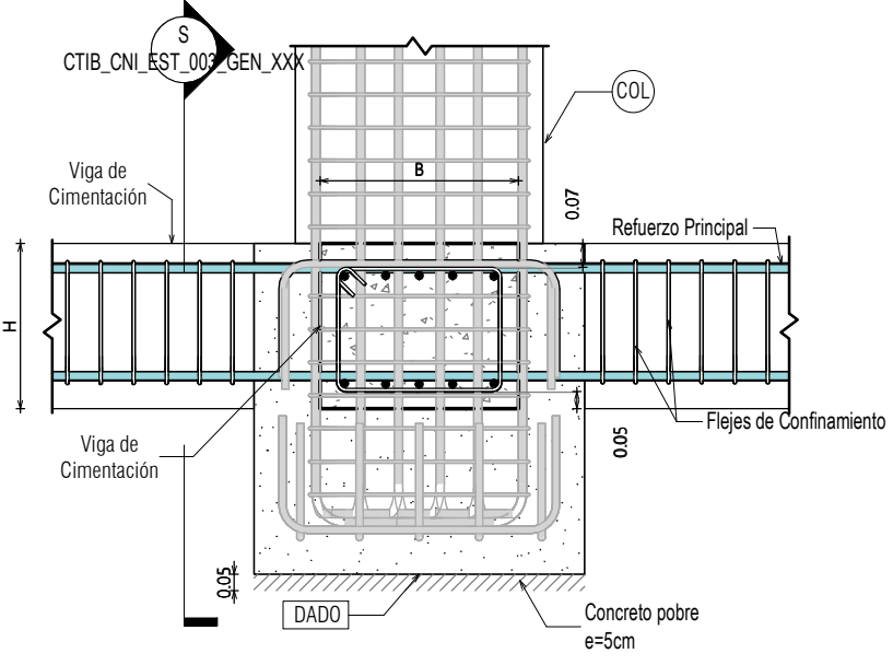
CORTE T-T
