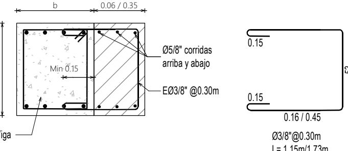
SECCIÓN TÍPICA DE SOBRECANTO escala 1 : 25
