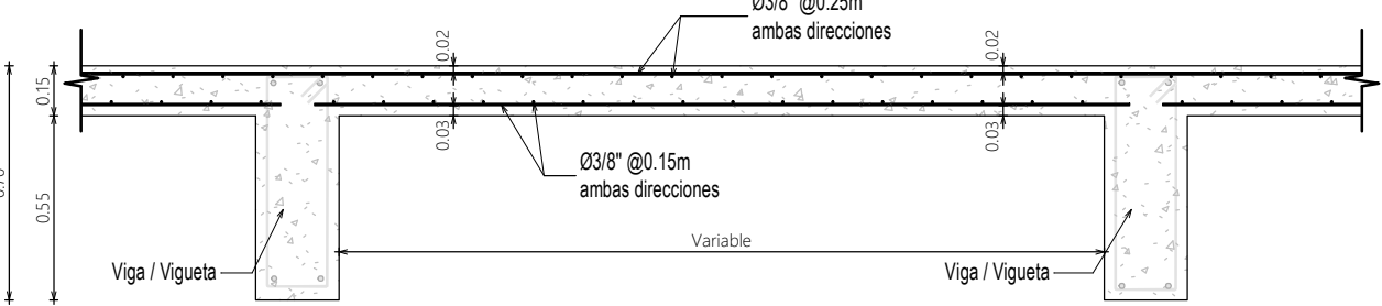
SECCIÓN TÍPICA DE PLACA e=15cm escala 1 : 25
