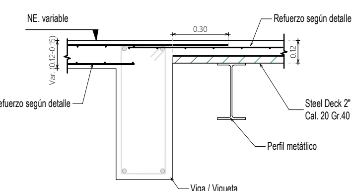
DETALLE TRANSICIÓN PLACA-STEELDECK escala 1 : 20
