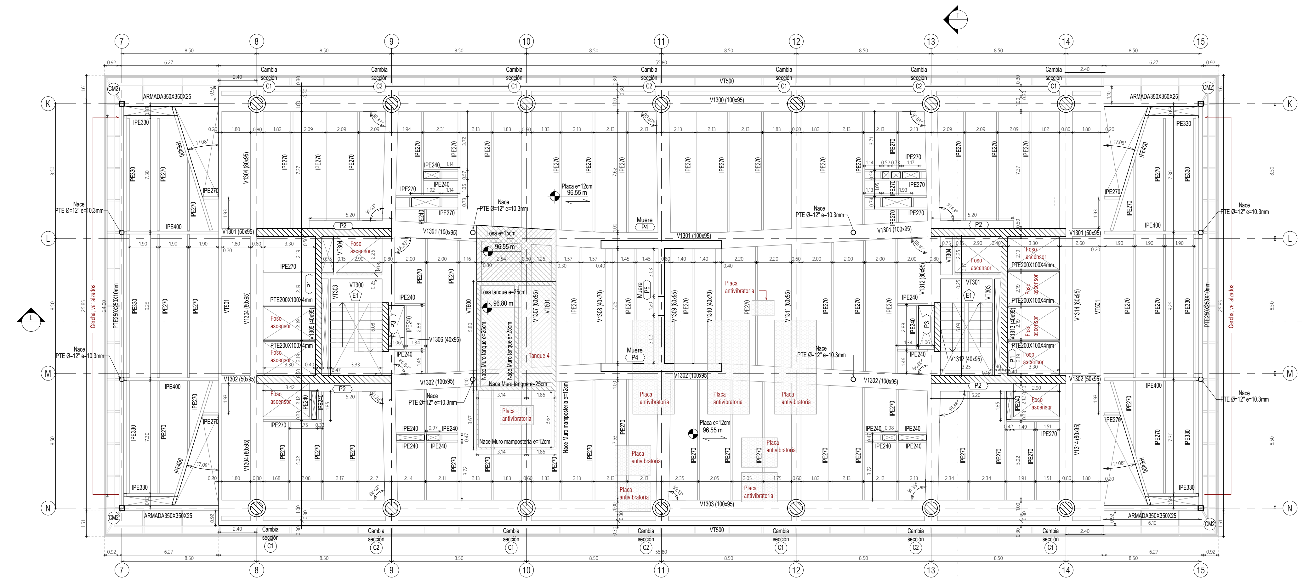
PLANTA DE N.E. TERRAZA N.E. +96.55m escala 1 : 150
