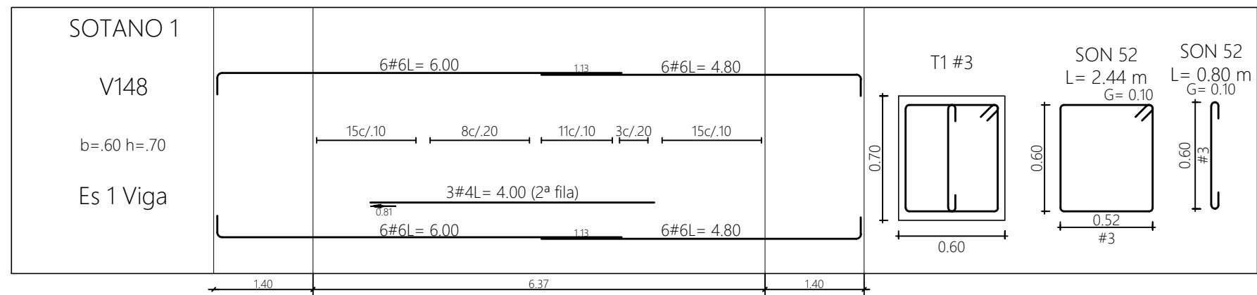
DESPIECE DE VIGAS SÓTANO 1 Escala 1:75
