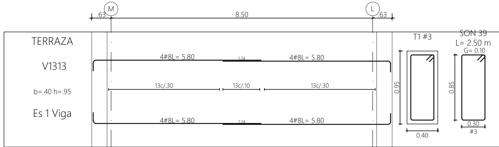
DESPIECES DE VIGAS DE TERRAZA escala 1:75
