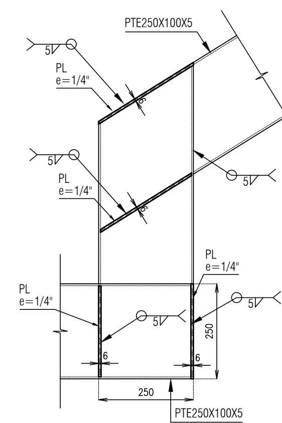
Detalle D5 escala 1:10
