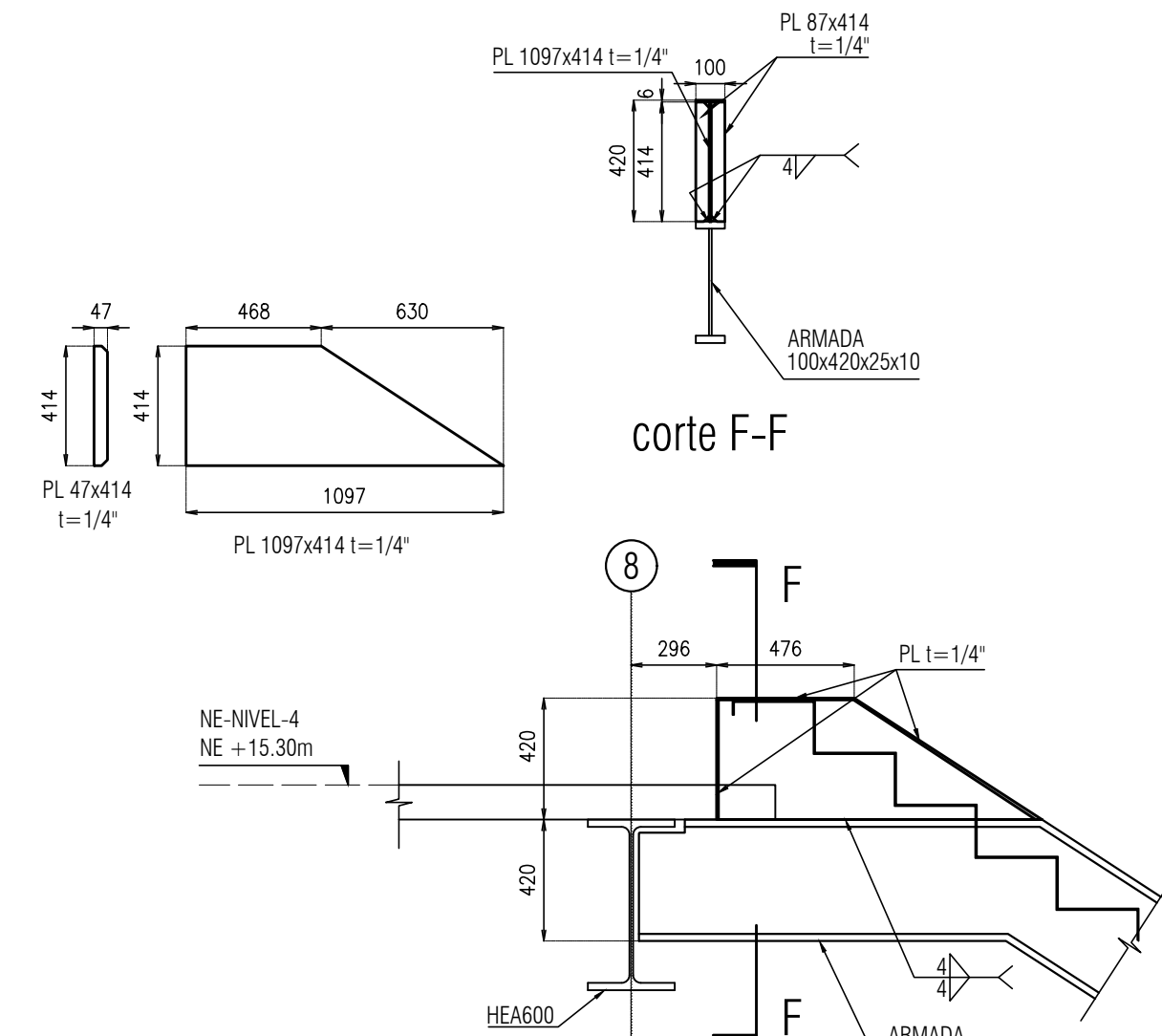
DETALLE D1 escala 1:25
