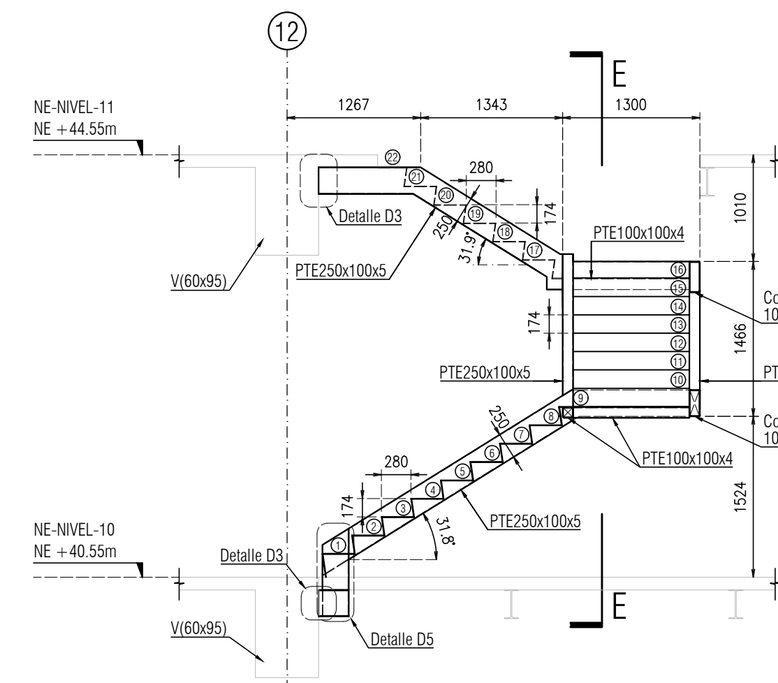
CORTE D - D ESCALERA E6 escala 1:50
