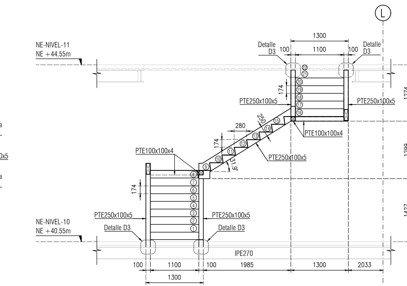
CORTE E - E ESCALERA E6 escala 1:50
