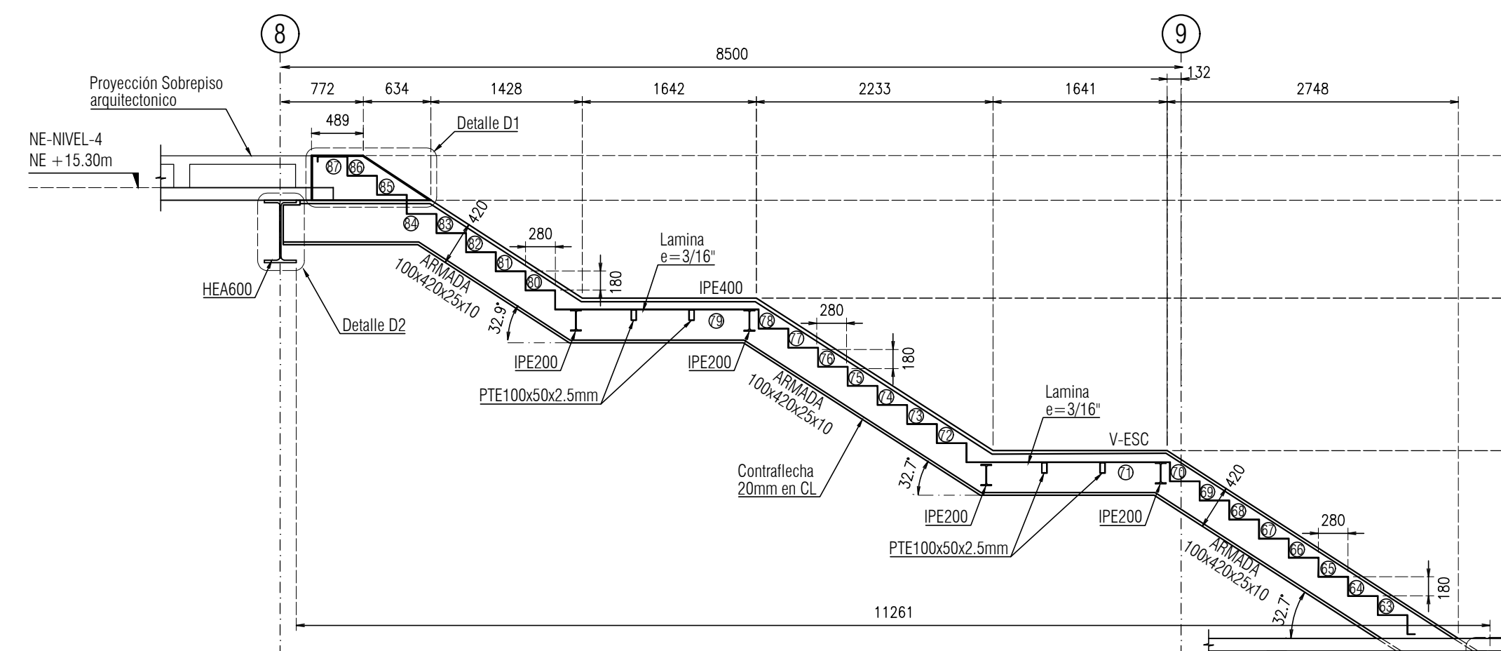
CORTE C - C ESCALERA E5 escala 1:50
