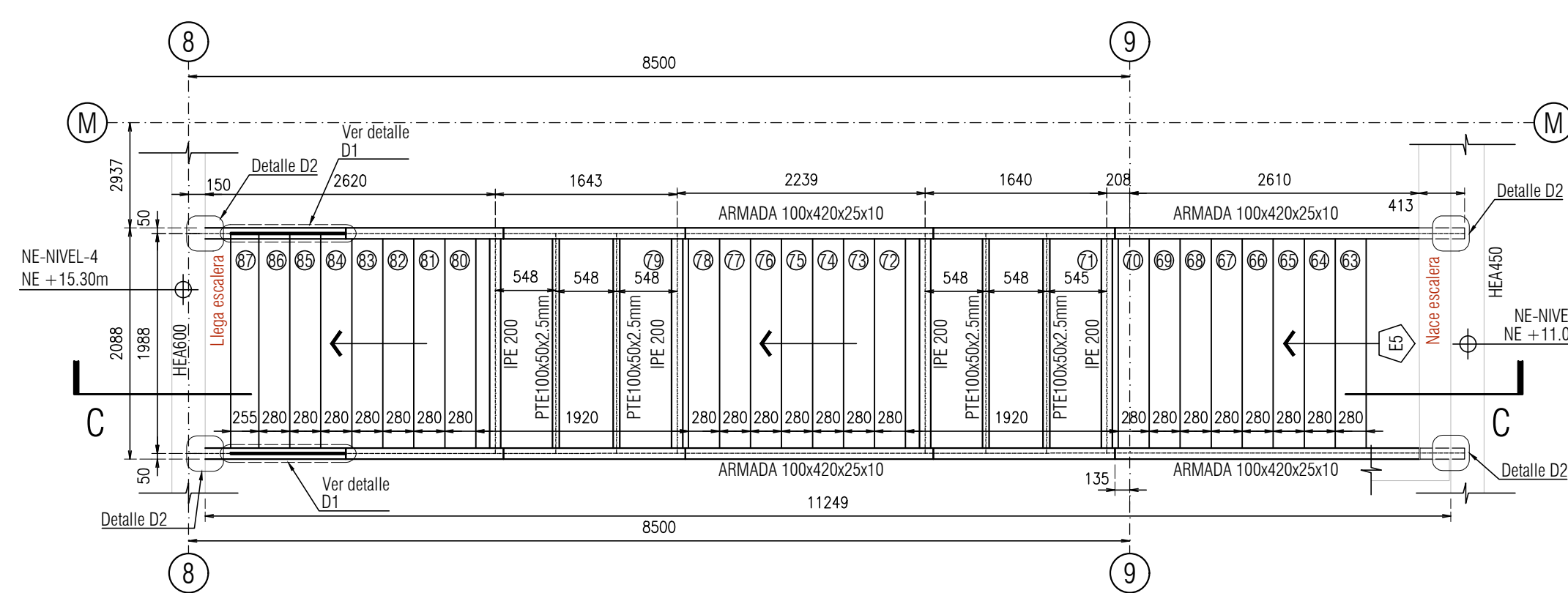
PLANTA ESCALERA E5 escala 1:50
