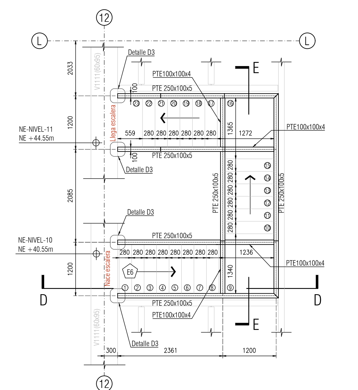
PLANTA ESCALERA E6 escala 1:50
