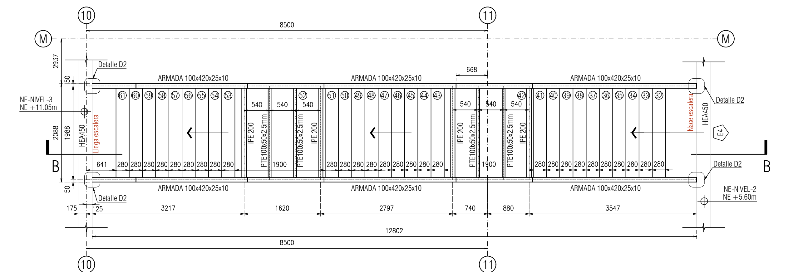
PLANTA ESCALERA E4 escala 1:50
