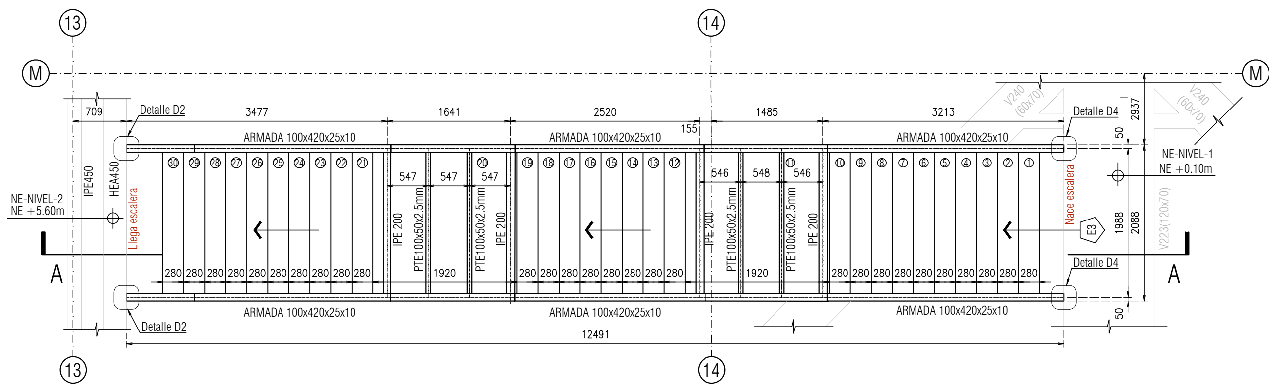
PLANTA ESCALERA E3 escala 1:50
