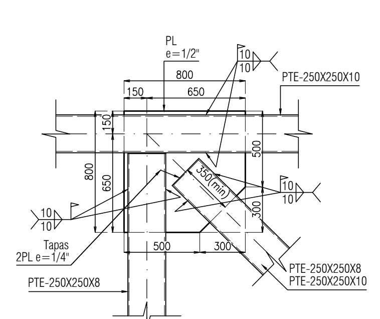
Detalle 15 escala 1:25
