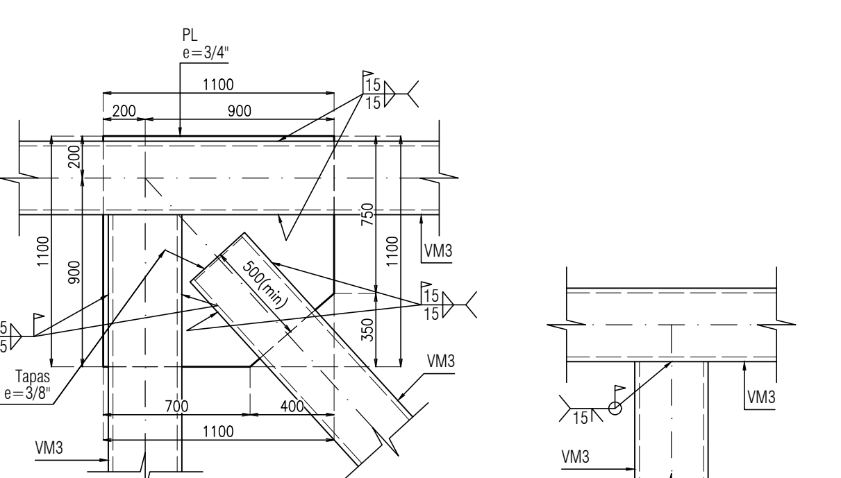
Detalle 12 escala 1:25
