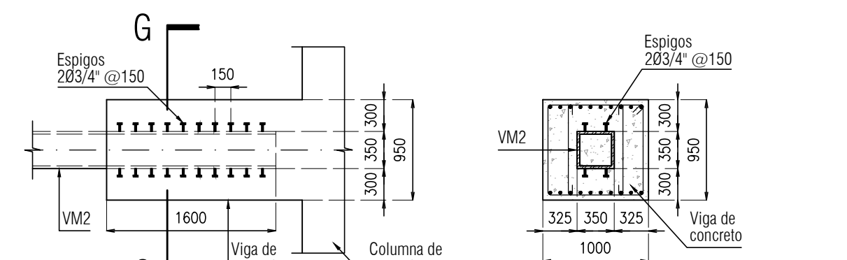
Detalle 21 escala 1:50
