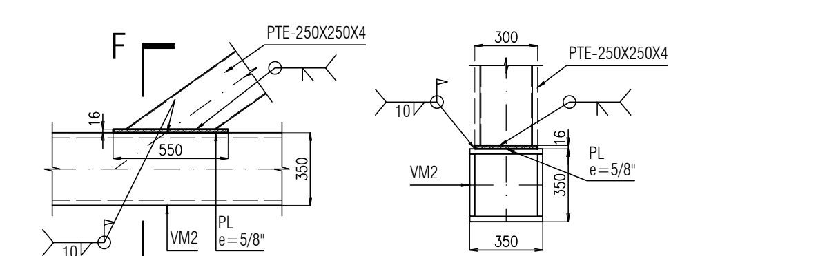
Detalle 20 escala 1:25
