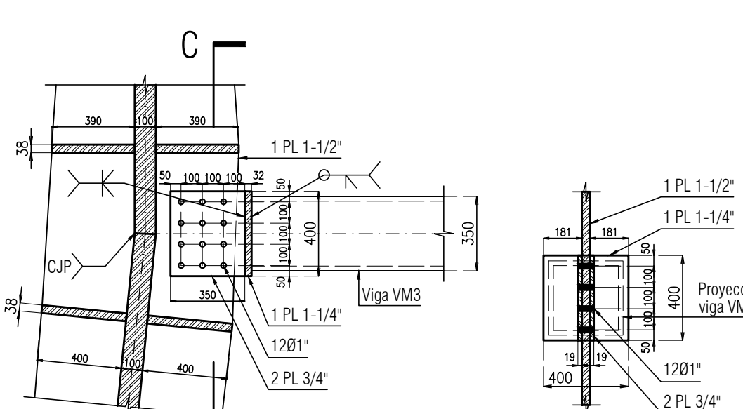
Detalle 1 escala 1:25
