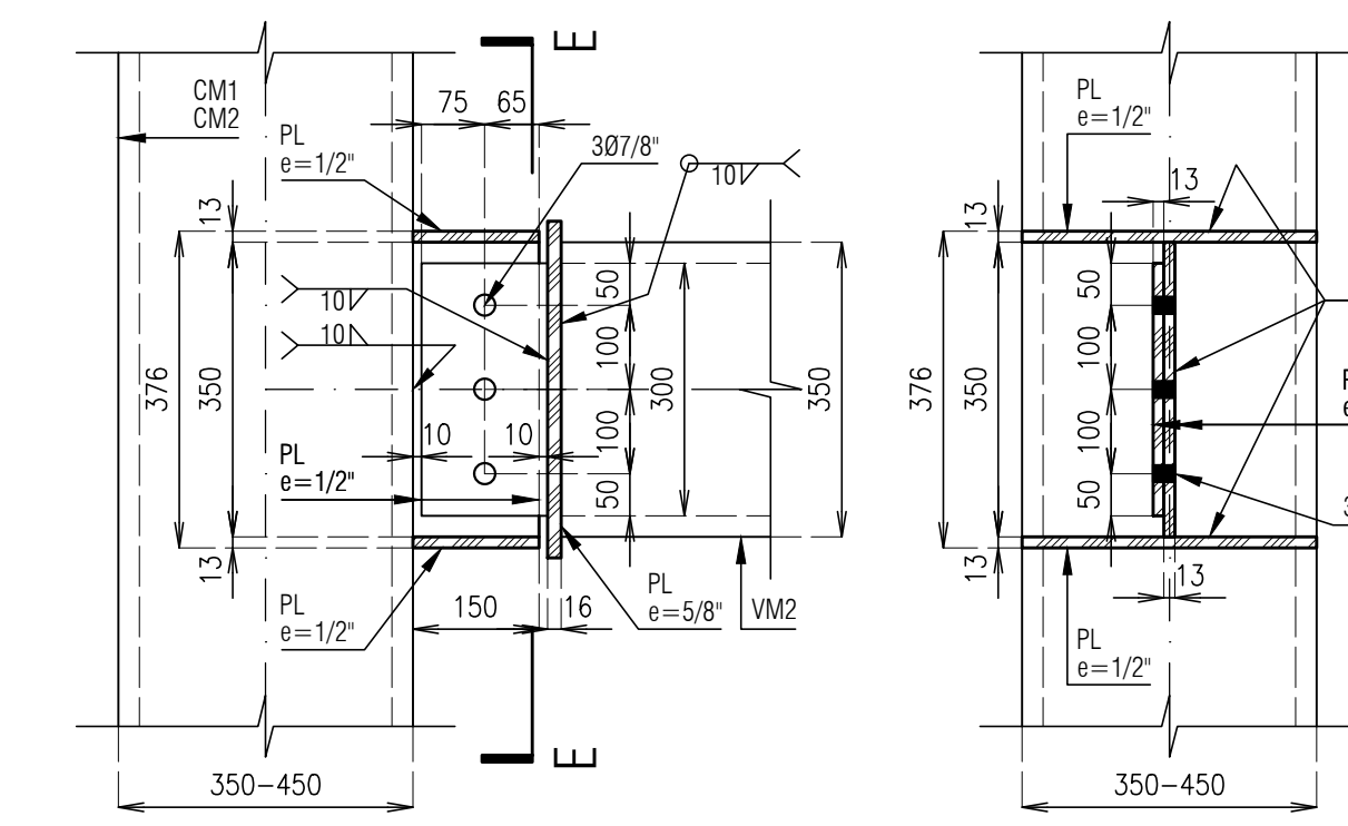
Detalle 19 escala 1:10
