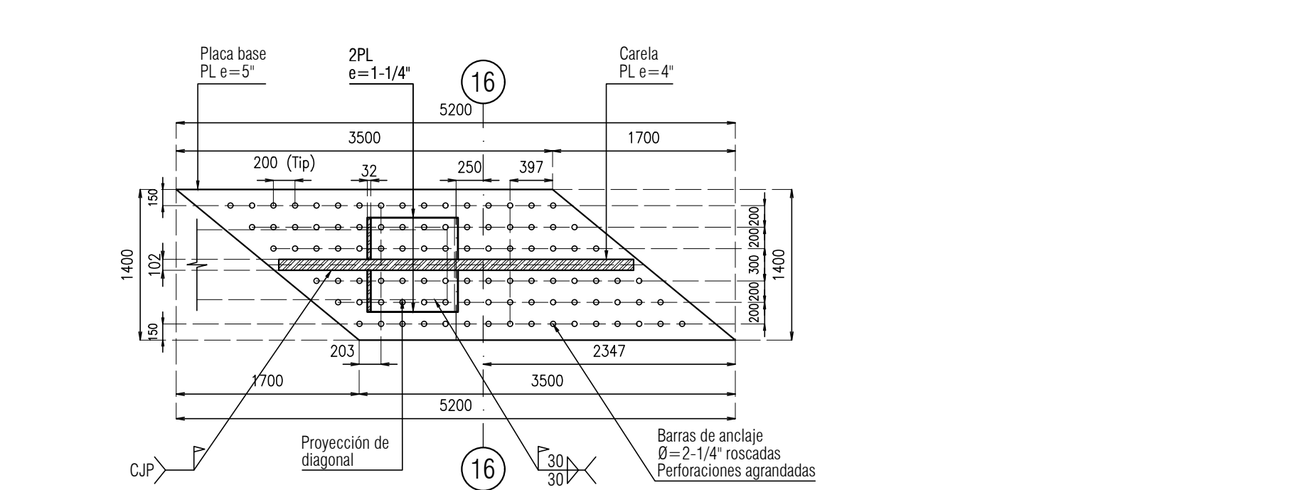
Detalle 2B escala 1:50
