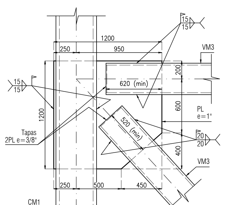
Detalle 9 escala 1:25
