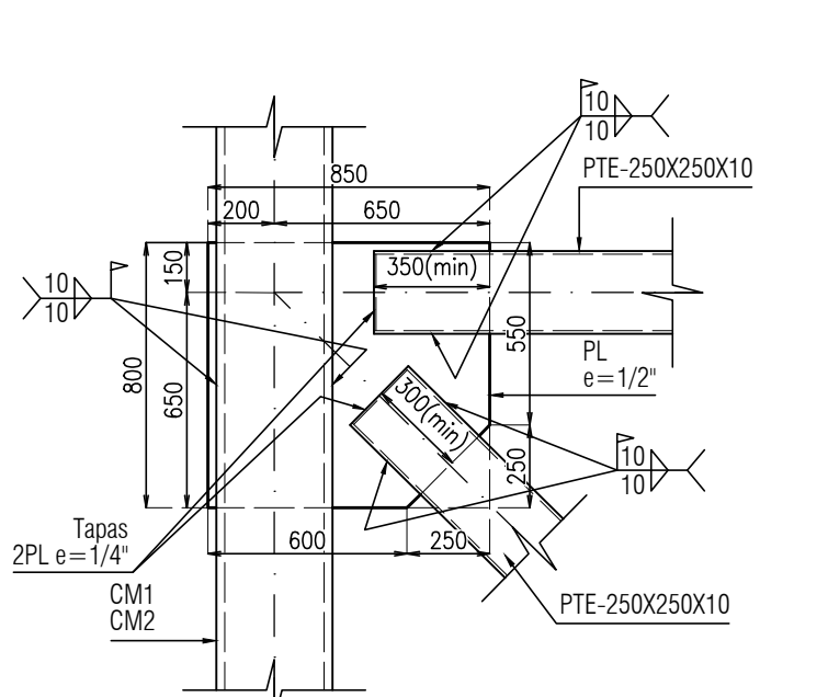
Detalle 14 escala 1:25
