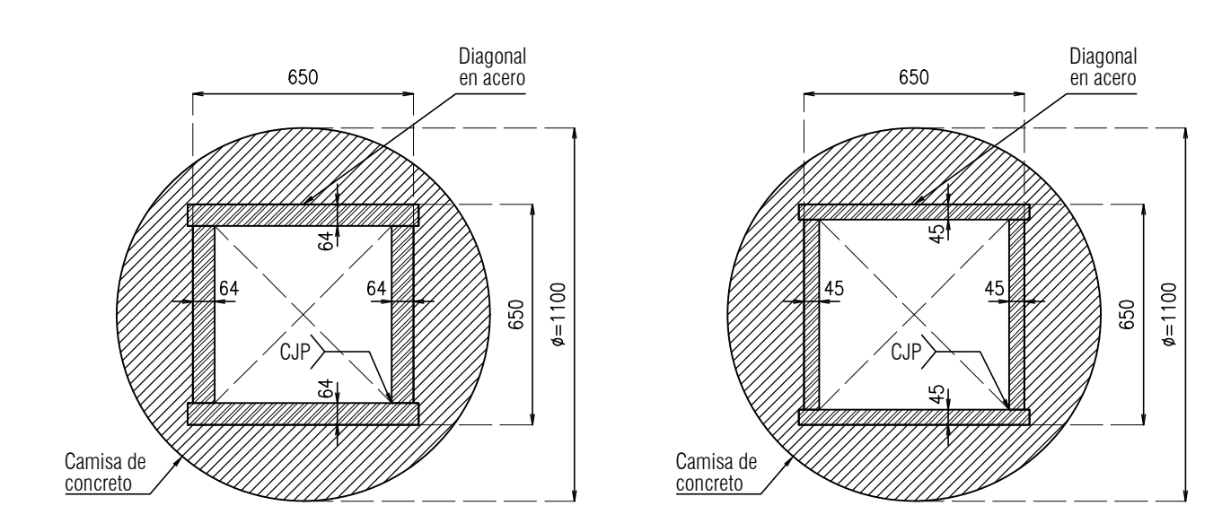
SECCION DIAGONAL D1 escala 1:20
