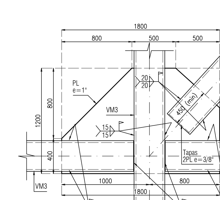
Detalle 10 escala 1:25
