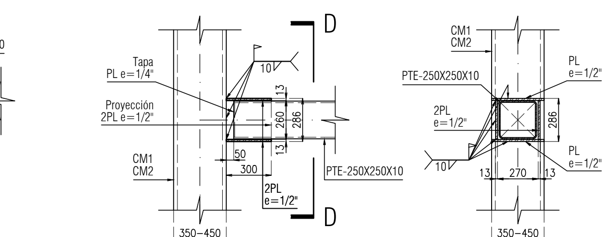
Detalle 18 escala 1:25
