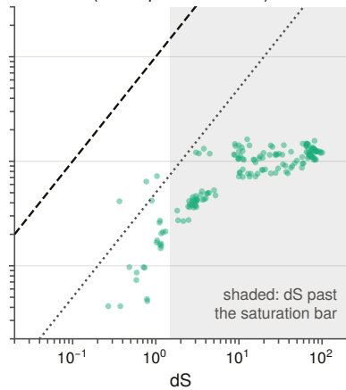
ITPR3 (85 % past dS = 1.5)
