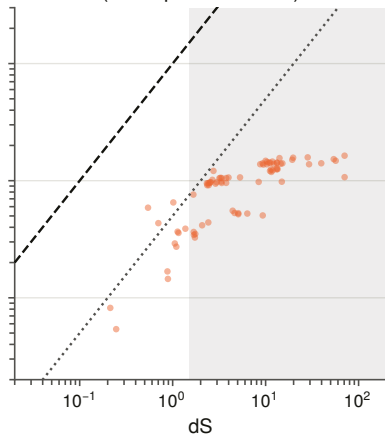
ITPR2 (85 % past dS = 1.5)
