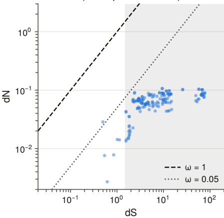
ITPR1 (94 % past dS = 1.5)
