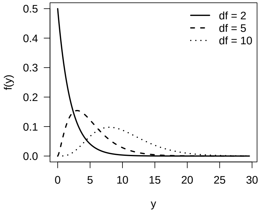
\chi^2 -distribution \chi^2(df)
