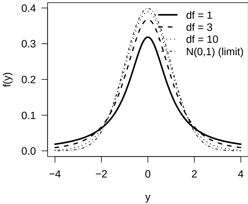
t-distribution t(df)
