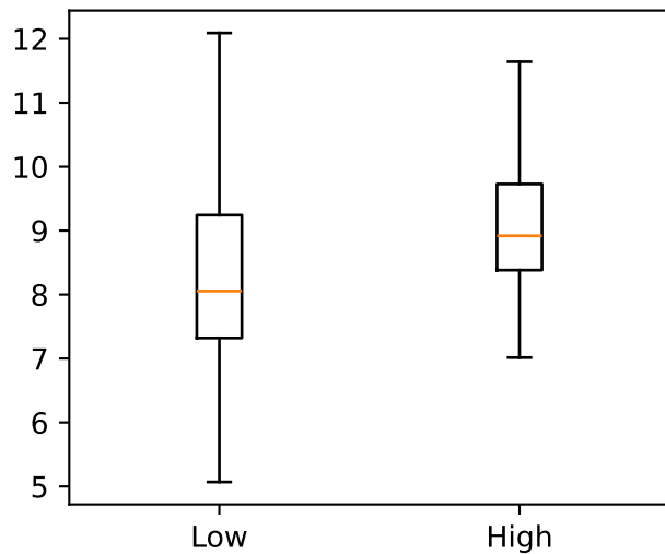
IDO1
