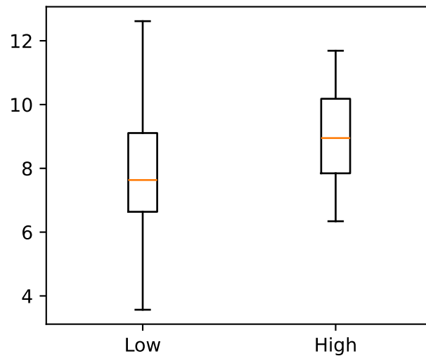
GZMB
