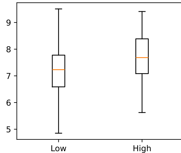
PRF1
