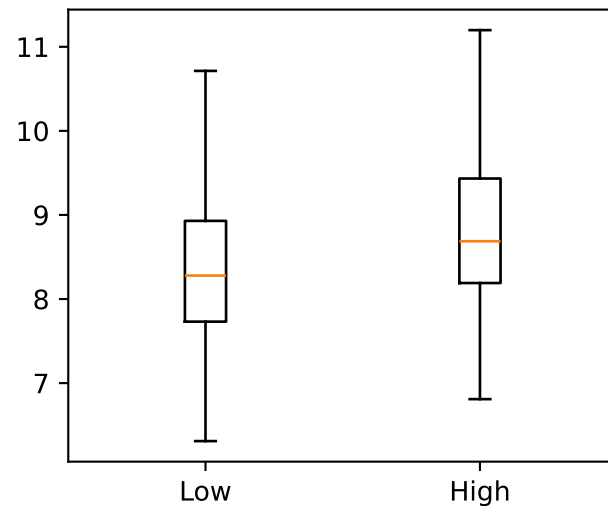
PRF1
