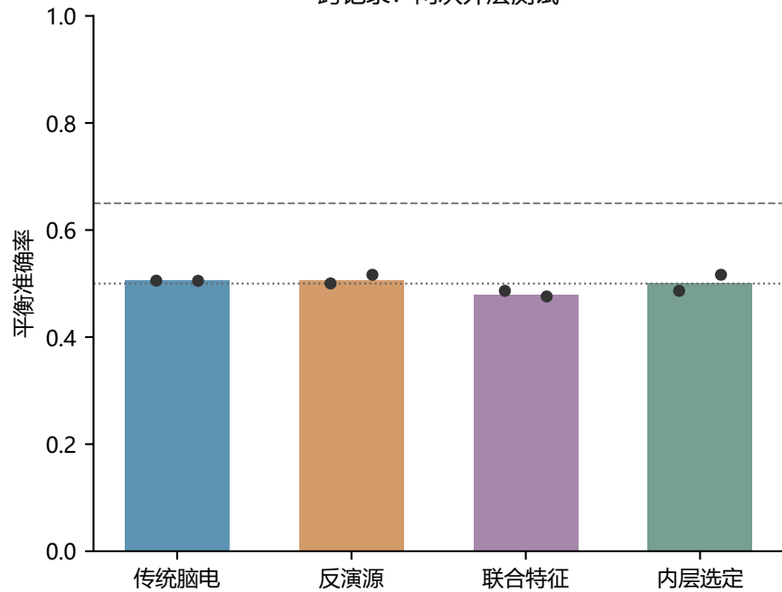
跨记录：两次外层测试
