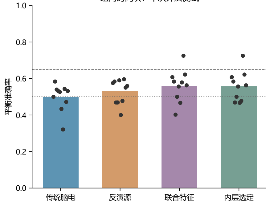
组内时间块：十次外层测试
