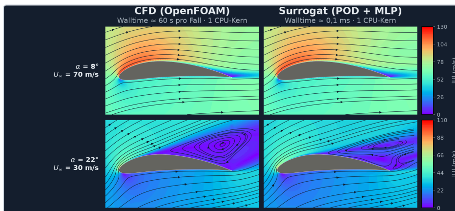
Geschwindigkeitsfeld |U| — CFD vs. Surrogat (POD + MLP) für die zwei Testfälle.
