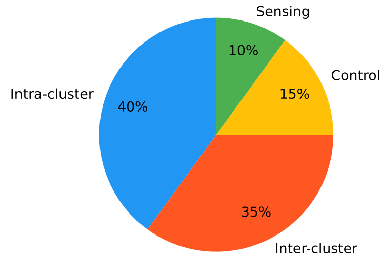
EERP
