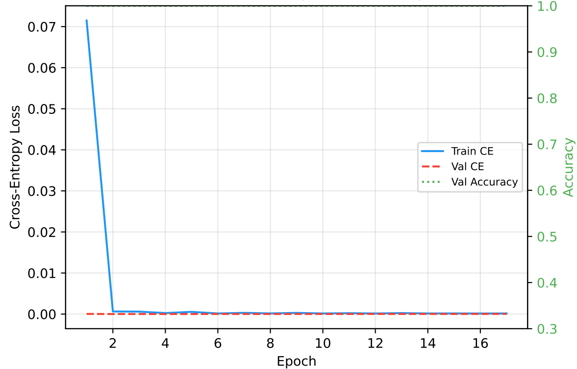
(d) GNN Encoder + Policy ( f_\theta, \pi_\theta , \sim 37K params)
